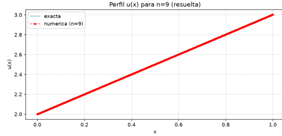
Figura 3: Perfil de u(x) para n = 9 ( M = 513 ): la onda queda bien resuelta.
