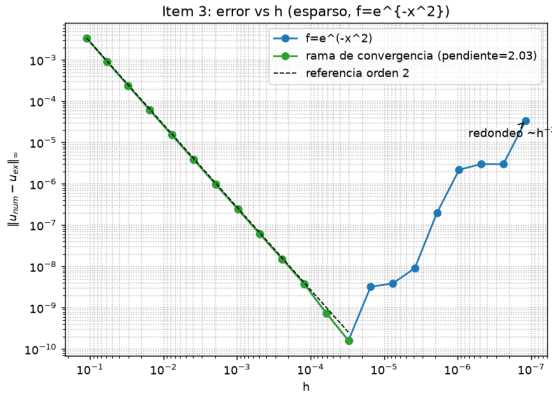
Figura 4: Orden 2 en la convergencia y subida por redondeo.
