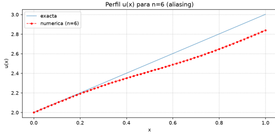
Figura 2: Perfil de u(x) para n = 6 ( M = 65 ): submuestreo severo y fallo por aliasing.
