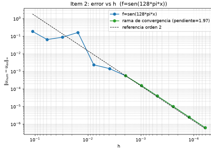
Figura 1: Error en norma infinito vs h para f = \text{sen}(128\pi x) . Orden 2 (pendiente \approx 1,97 ) visible una vez superado el aliasing de la alta frecuencia.
