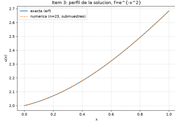
Figura 5: Perfil u(x) para n = 23 (submuestreado para graficar).
