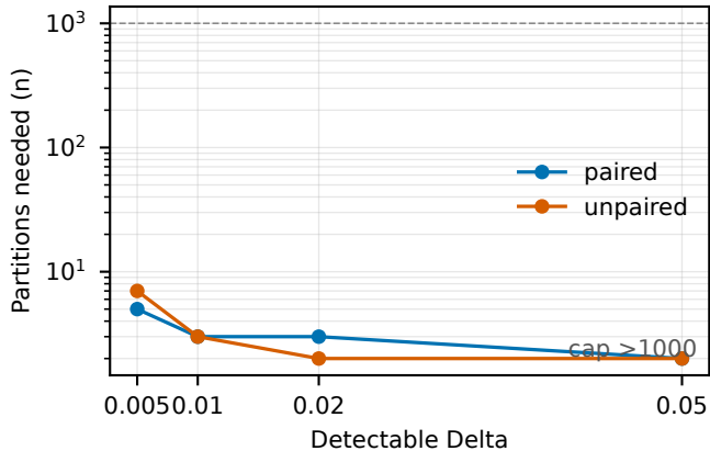
TinyLlama-1.1B
