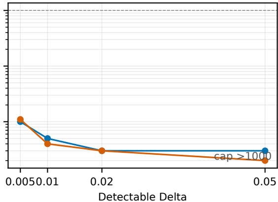
LLaMA-3.2-3B
