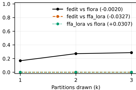
LLaMA-3.2-3B: per-pair (paired)
