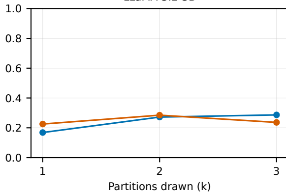
LLaMA-3.2-3B
