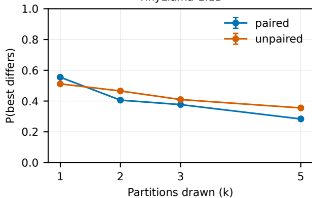
TinyLlama-1.1B
