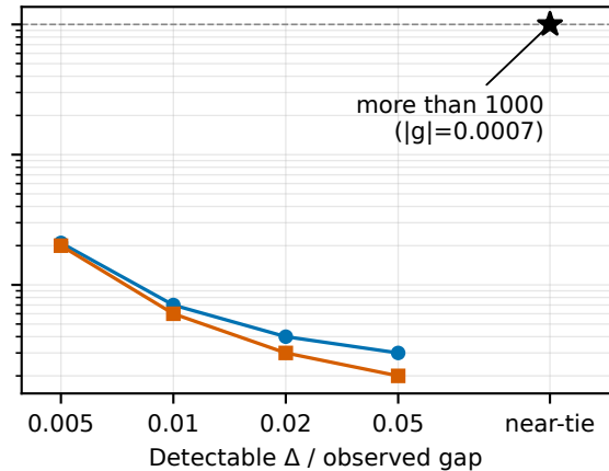
LLaMA-3.2-3B ( p = 10 )
