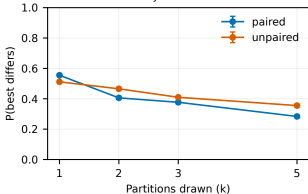
TinyLlama-1.1B
