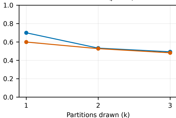
LLaMA-3.2-3B ( p = 10 )
