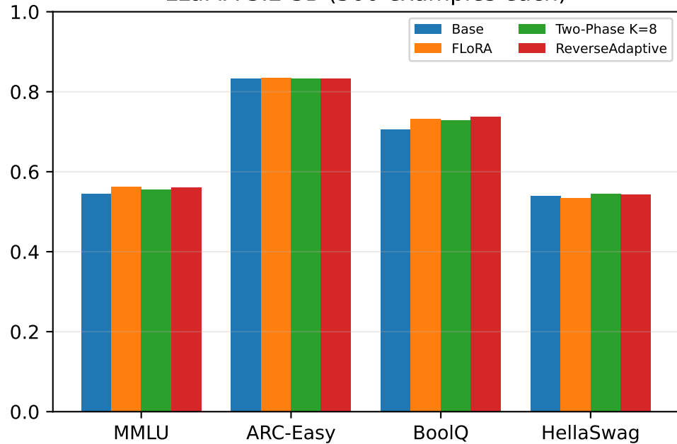
LLaMA-3.2-3B (500 examples each)
