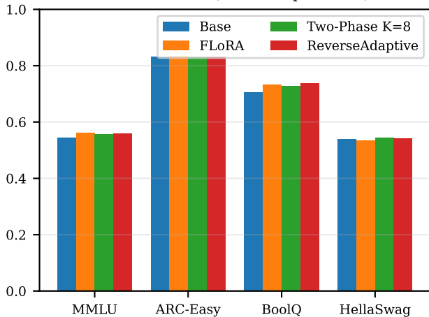
LLaMA-3.2-3B (500 examples each)
