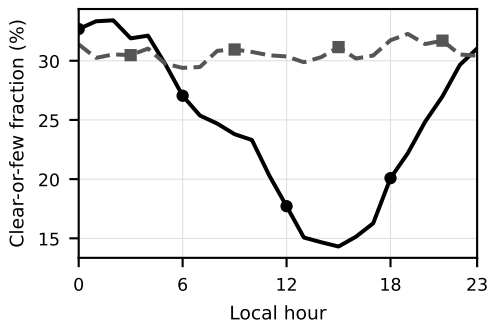
(d) Toronto: human vs. automated
