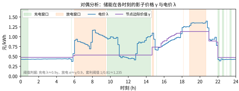
图 2: 储能节点边际价值 \gamma 与电价 \lambda 的全天对比
