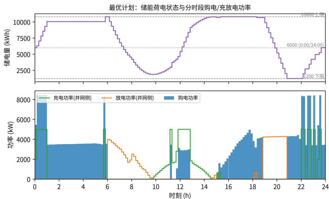
图 1: 解的储能状态与各时段购电、充电及放电功率
