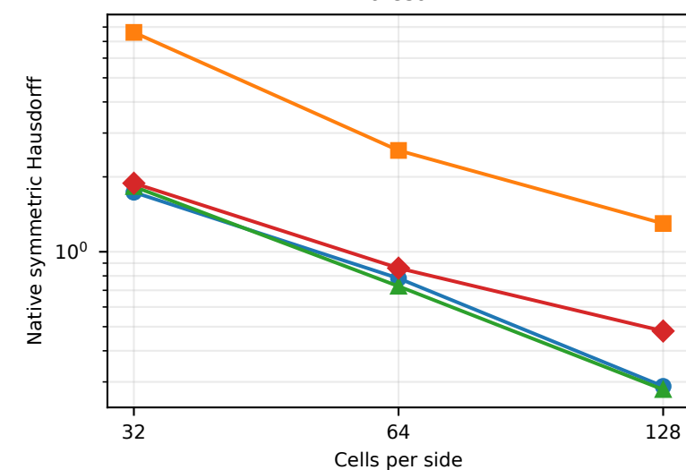
Zalesak
