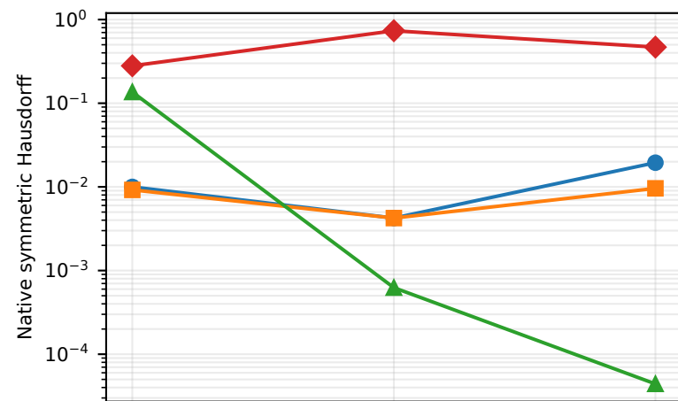
Zalesak
