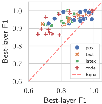
ERNIE-4.5-21B-A3B | Llama-3.2-3B
