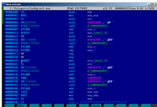
Figura 7.13: Hiew: JNZ NOPreemplazando JNZ con dos NOPs
