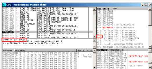
Figura 19.10: OllyDbg: i = 4 , (ZF =0)
