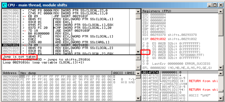
Figura 19.10: OllyDbg: i = 4 , (ZF = 0)
