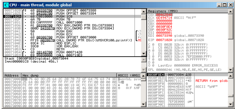
Figura 10.1: OllyDbg: se pasan las direcciones de dos variables globales a f1( )
