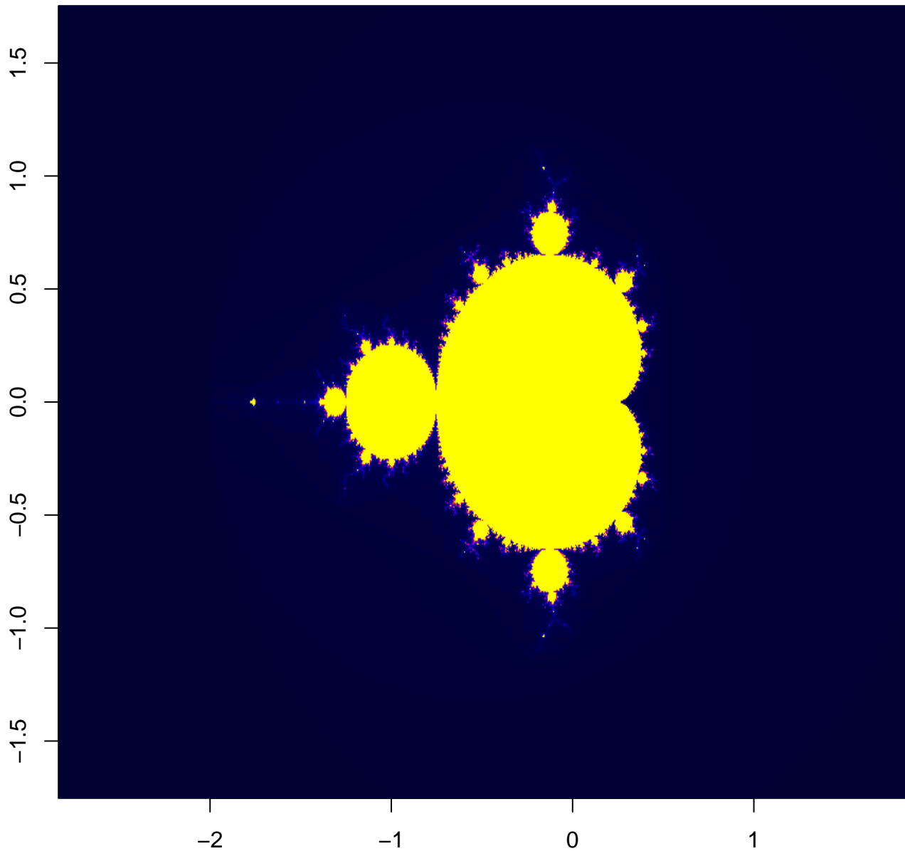
Mandelbrot Set (Zoom: 1.0x)
