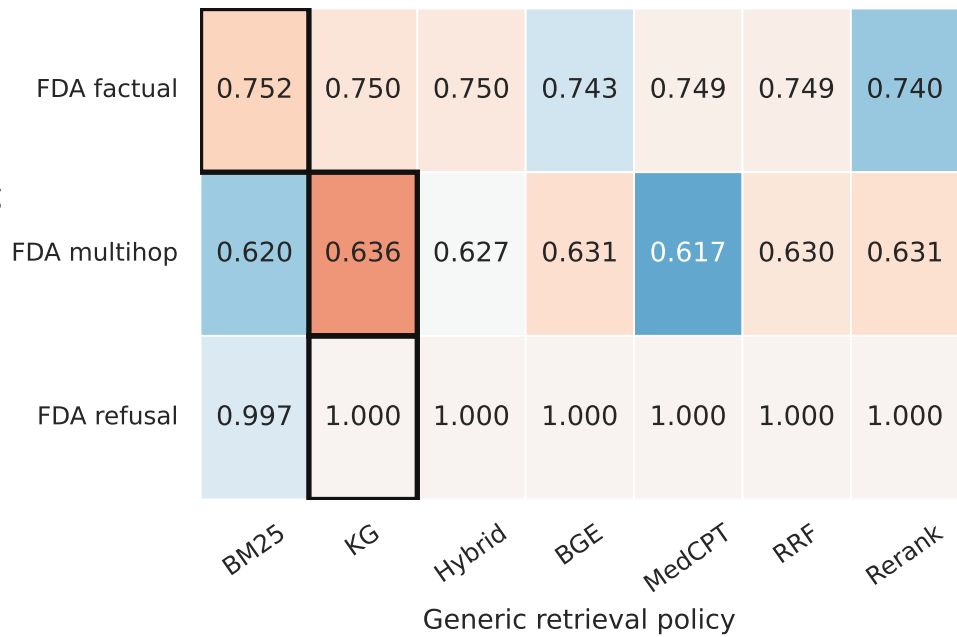
FDARxBench
