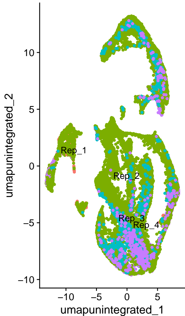
rep_group
