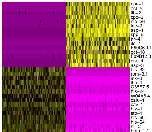
PC_1
