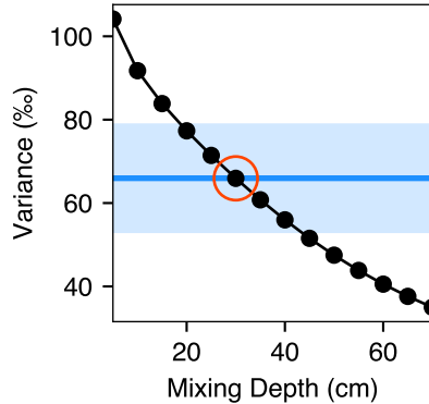
b. \delta^2\text{H}_{ice}
