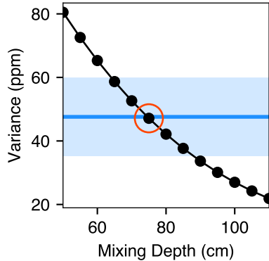
a. CO 2
