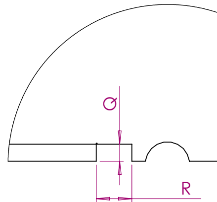
DETALLE A X4
