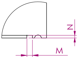
DETALLE A TYP X4 ESCALA 1 : 2
