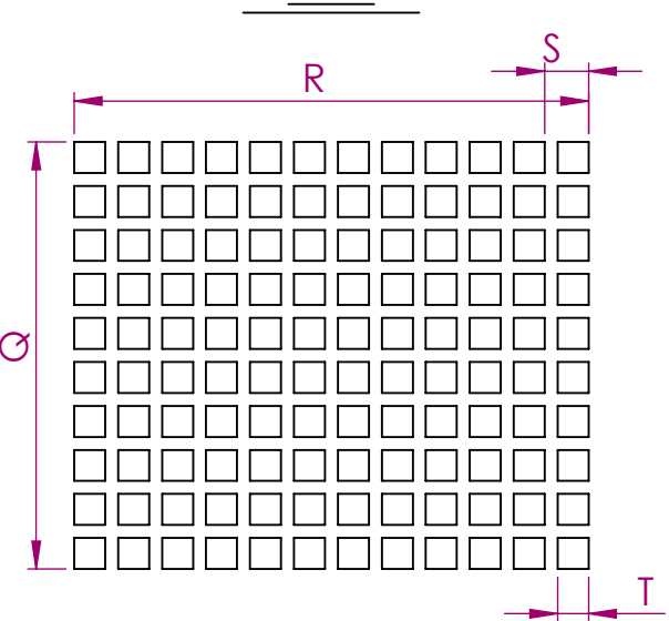
DETALLE B ESCALA 1 : 3
