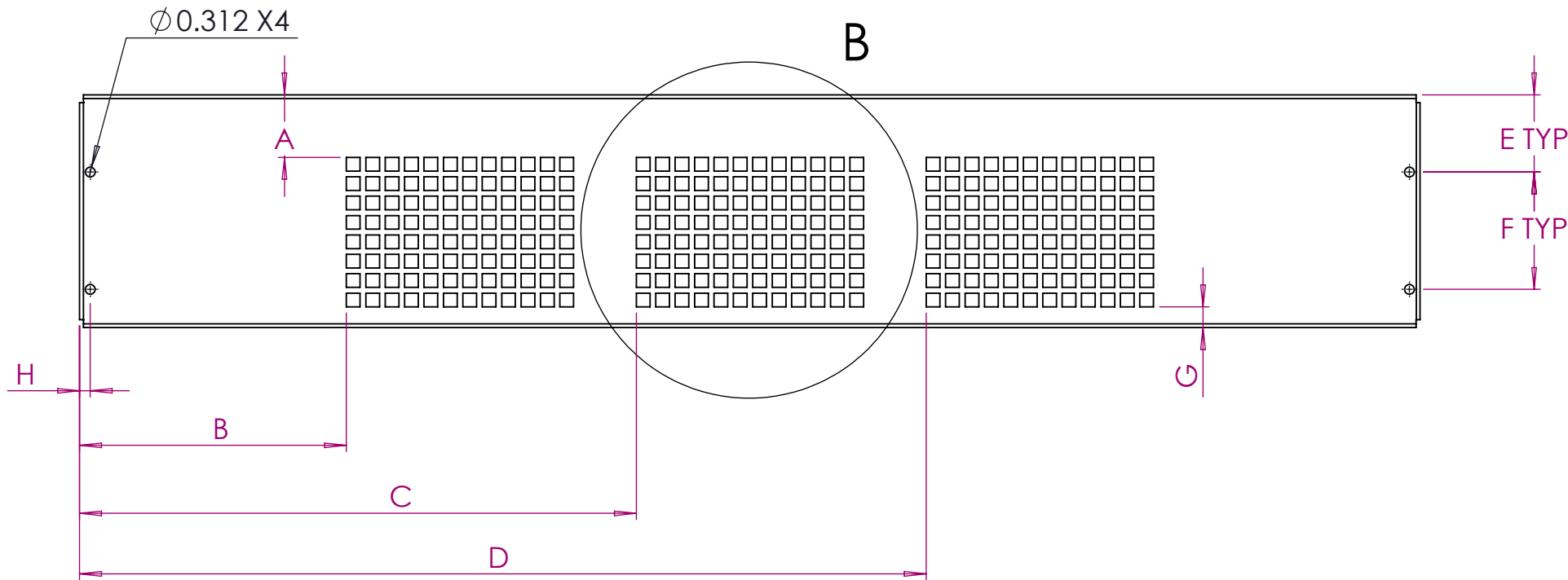
DETALLE B
