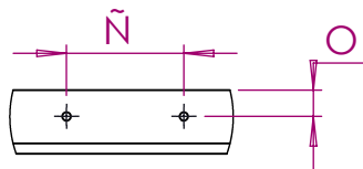
DETALLE A
