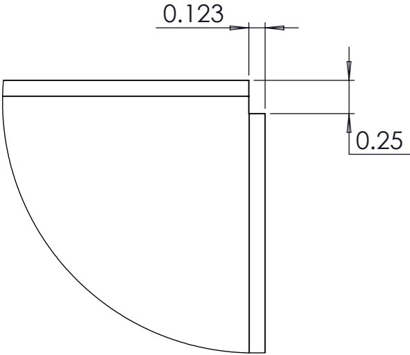
DETALLE A
