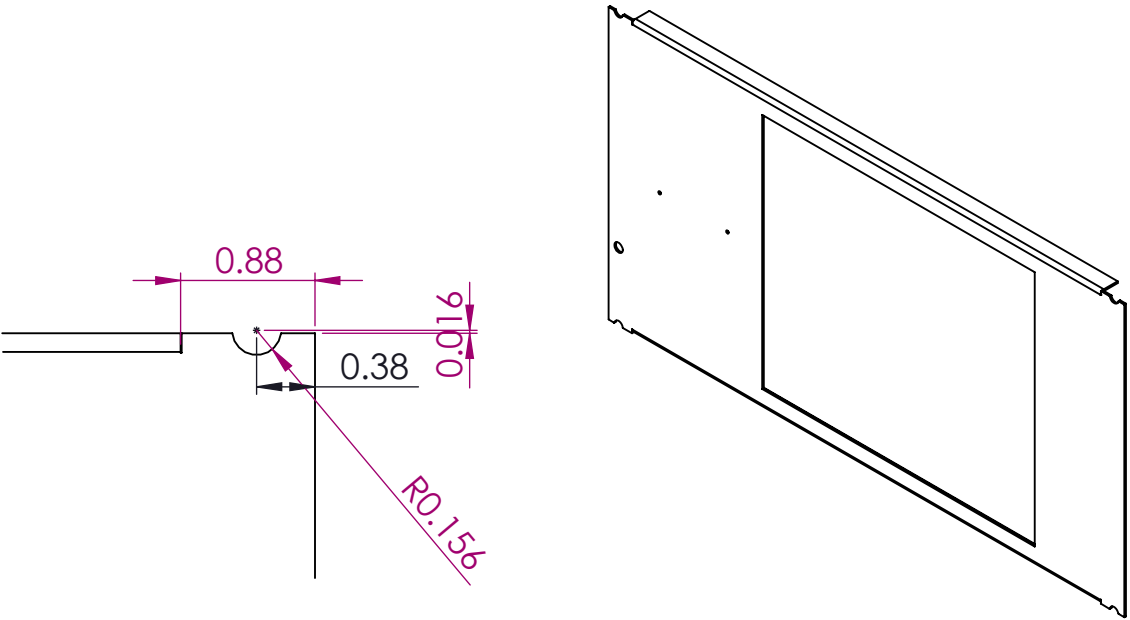
DETALLE A ESCALA 2 : 2.5
