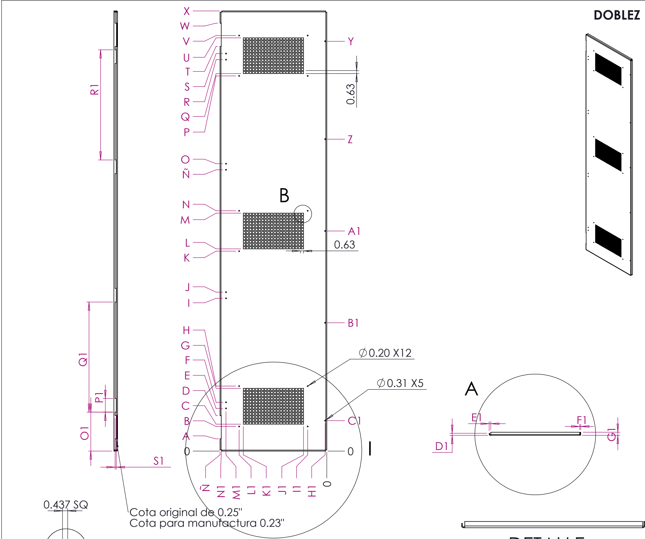
DETALLE A ESCALA 1 : 7
