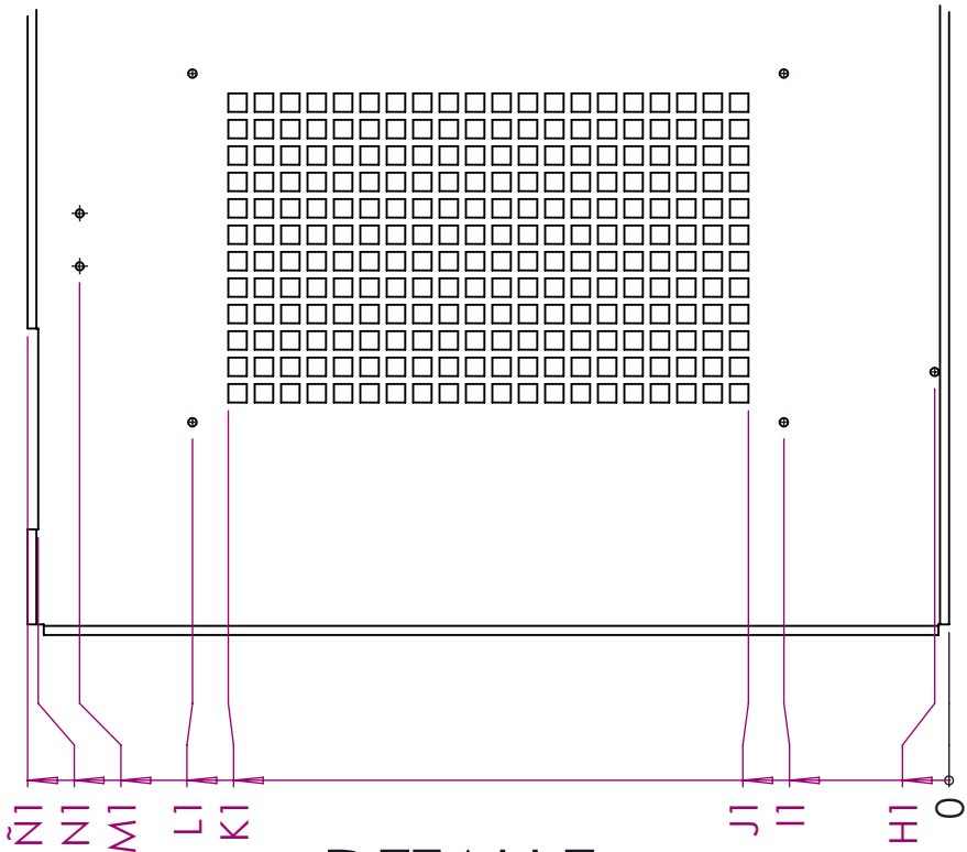
DETALLE J ESCALA 1 : 5
