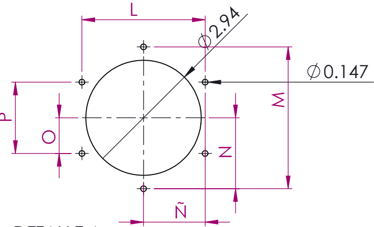
DETALLE A ESCALA 2 : 5
