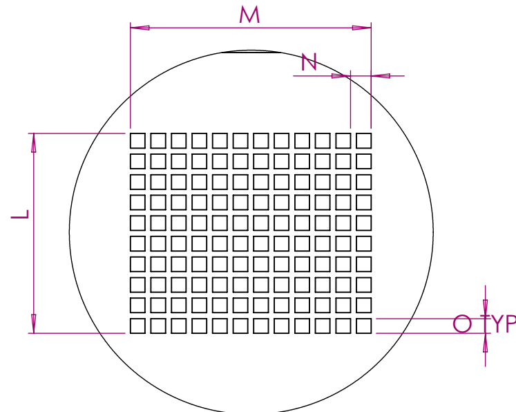
DETALLE A ESCALA 1 : 4
