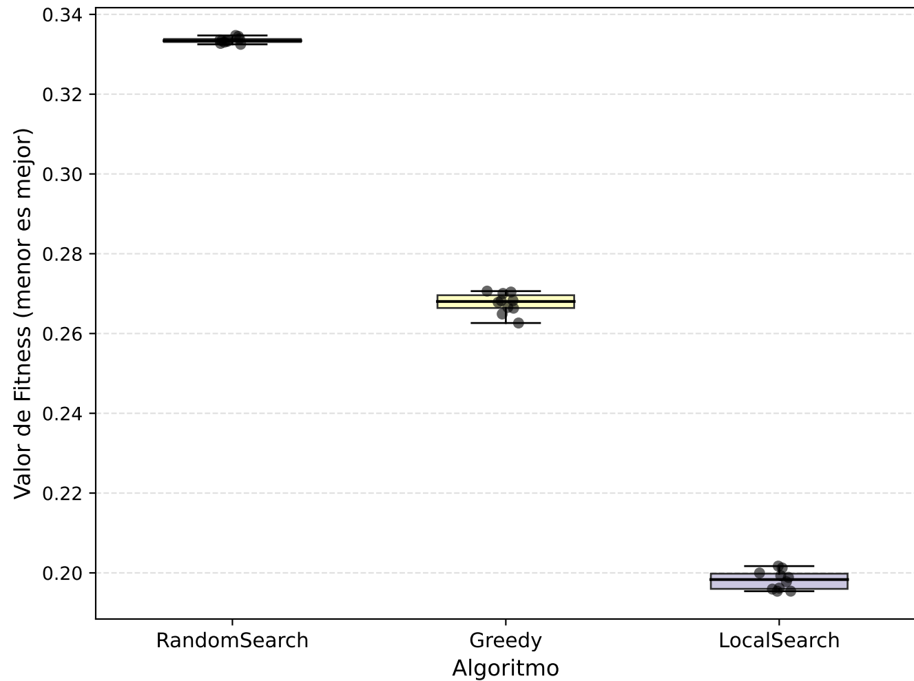
Distribución del Fitness - Dataset Bupa (30%)
