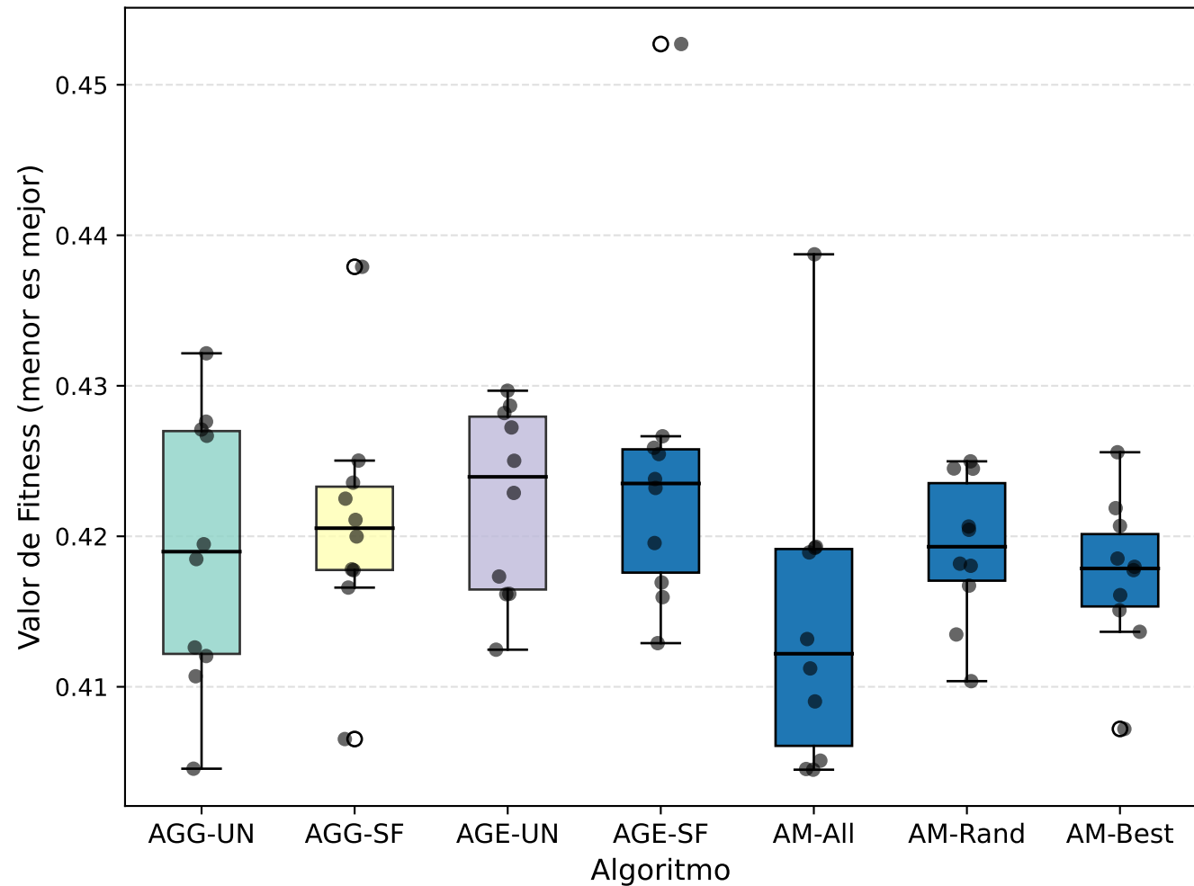
Distribución del Fitness - Dataset Glass (15%)
