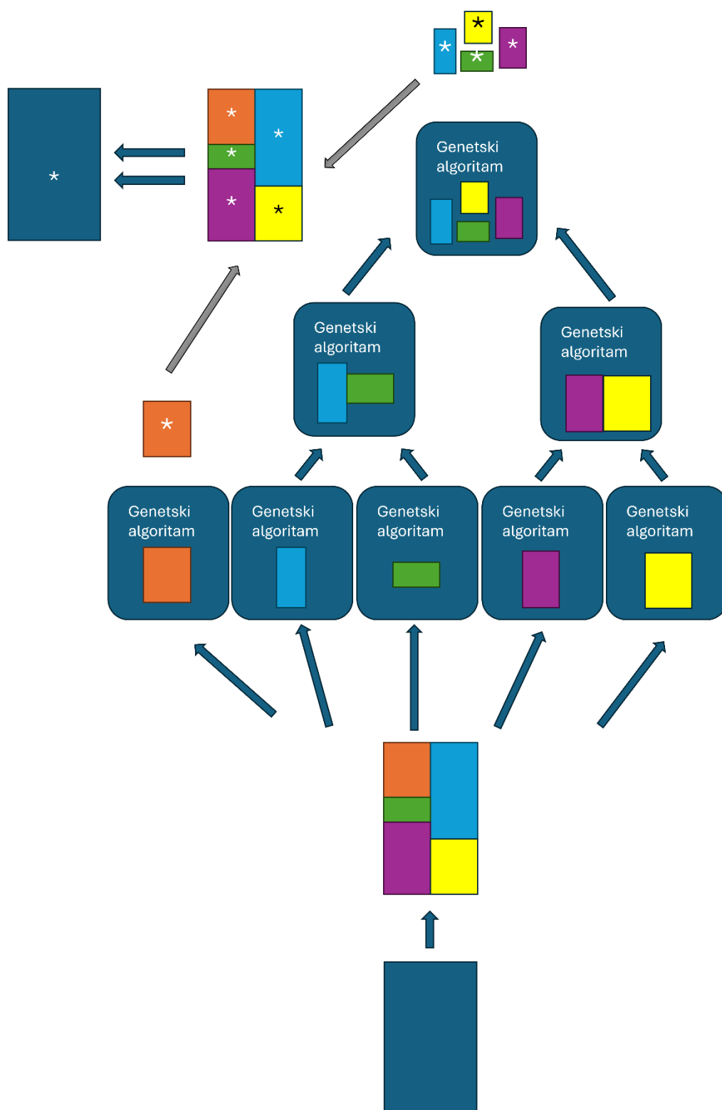
Slika 5 - prikaz procedure orkestriranog genetskog algoritma (početak odozdo)
