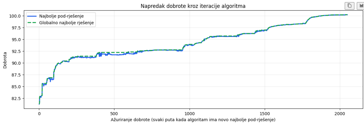
Slika 23 - dijagram napretka dobrote kroz iteracije algoritma za osječko-baranjsku županiju
