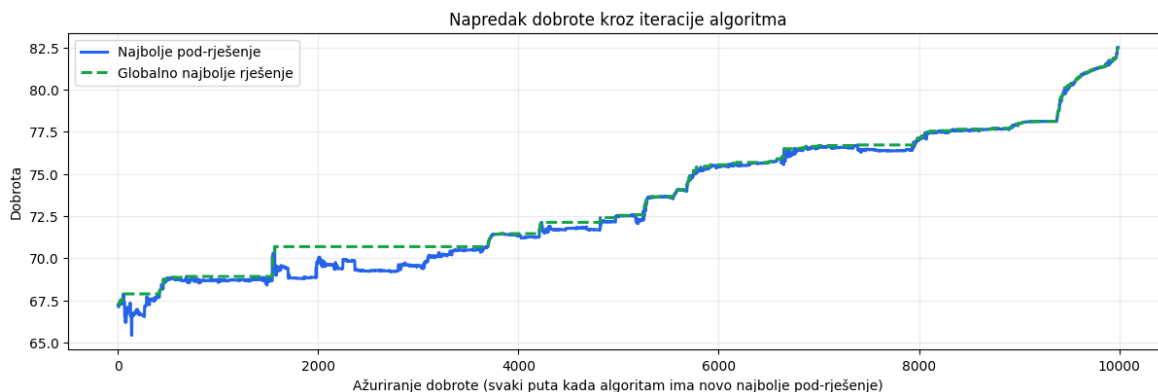
Slika 21 - dijagram napretka dobrote kroz iteracije algoritma za grad Zagreb
