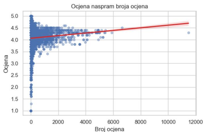
Slika 2 – linearna regresija ocjene naspram broja ocjena
