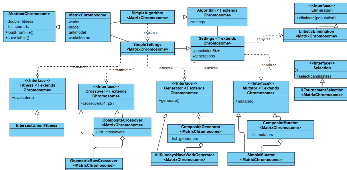
Slika 4 - dijagram klasa implementacije genetskog algoritma
