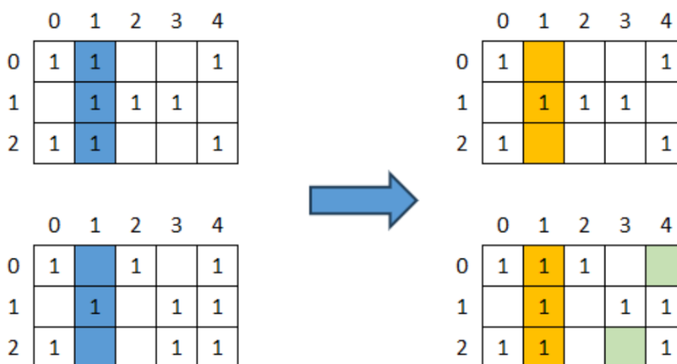
Slika 8 - dijagram križanja s k izmjena stupaca
