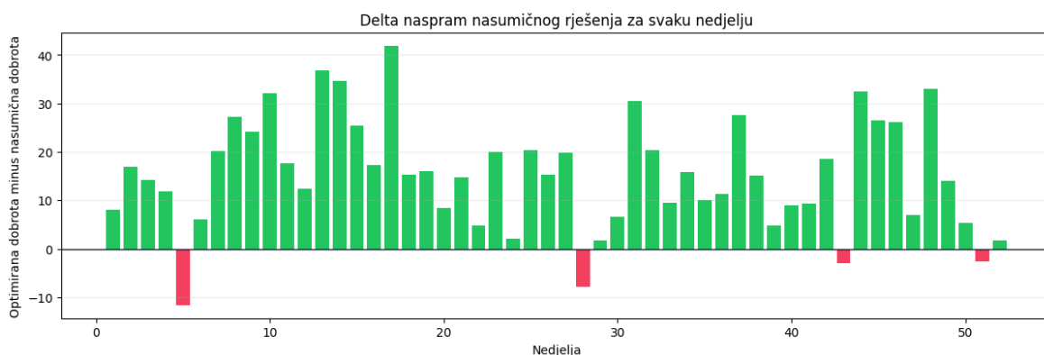
Slika 22 - dijagram promjene dobrote naspram nekog nasumičnog rješenja za svaku nedjelju
