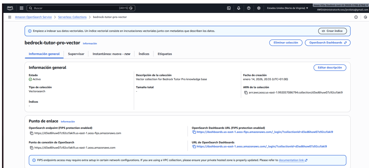
Figura 6: Finalización de la configuración de acceso y políticas de seguridad para la colección vectorial, asegurando la conectividad entre el motor de búsqueda y el orquestador de Bedrock.
