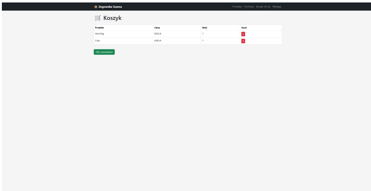
Rysunek 5. Koszyk
