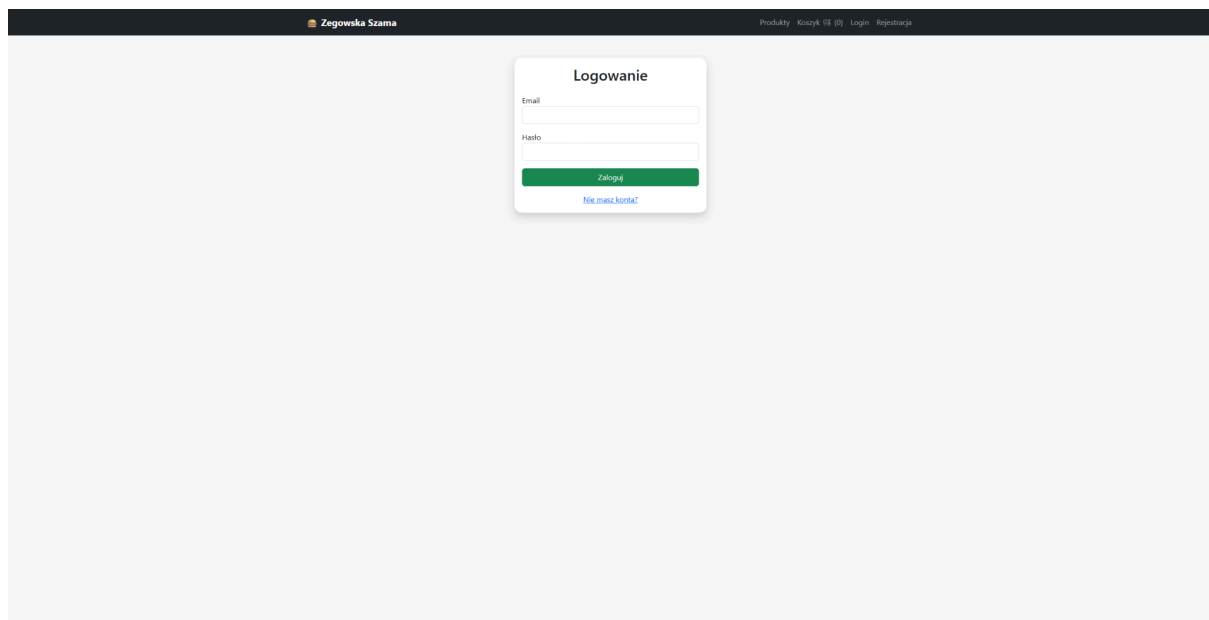
Rysunek 3. Logowanie
