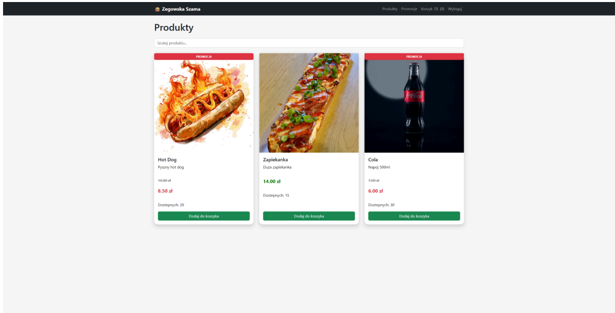
Rysunek 4. Produkty
