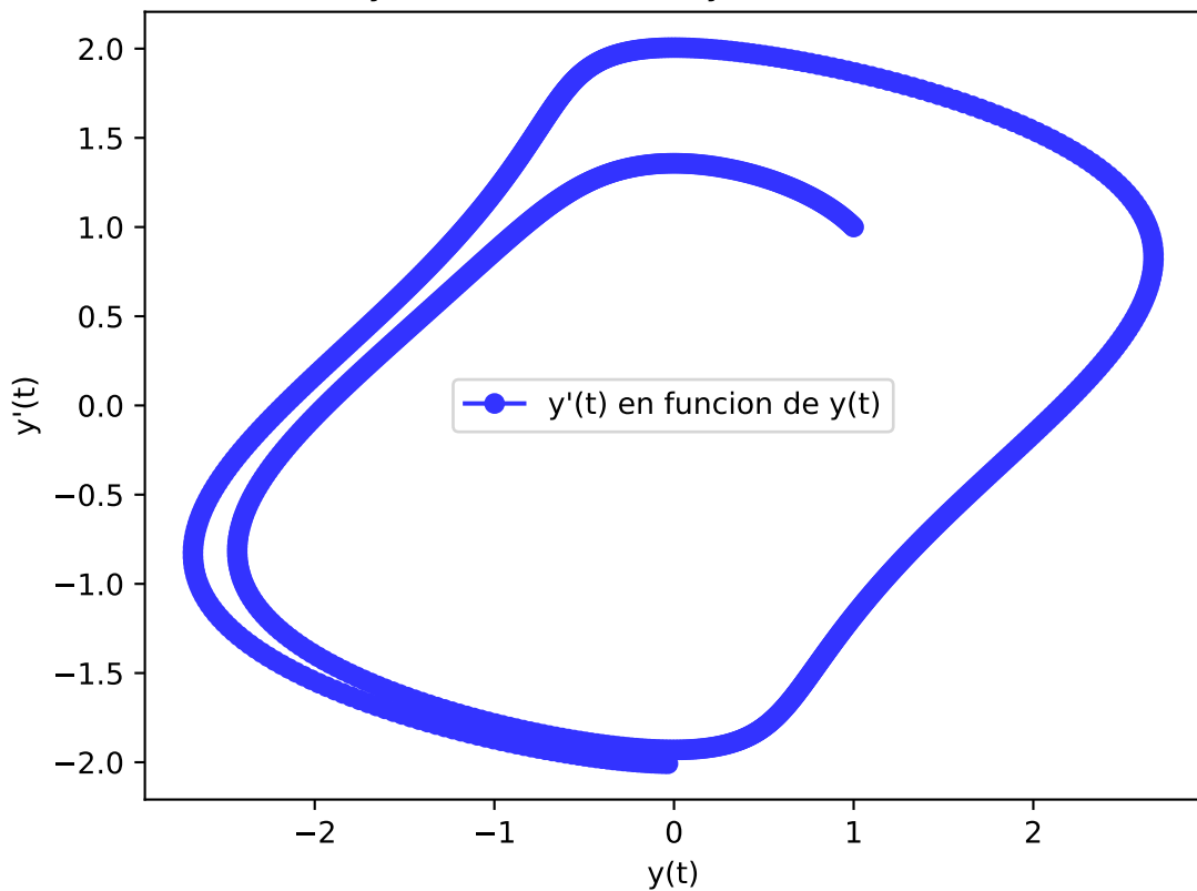
y'(t) en funcion de y(t) usando rk4
