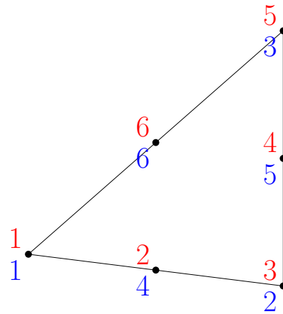
TRI6
