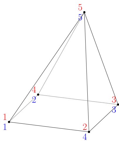
PYRA5
