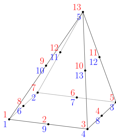
PYRA13
