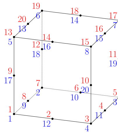
HEXA20
