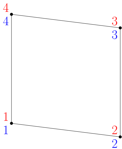
QUAD4
