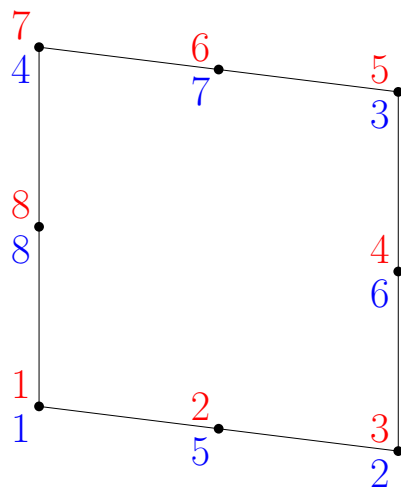
QUAD8
