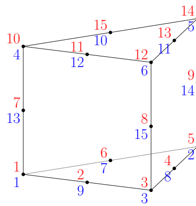
PENTA15
