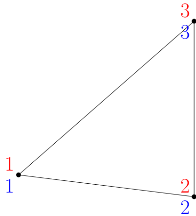
TRI3
