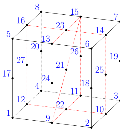
HEXA27
