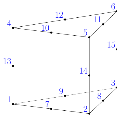
PENTA15
