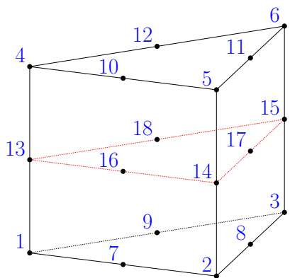
PENTA18
