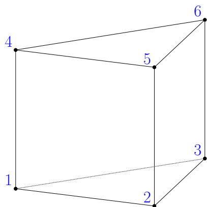
PENTA6
