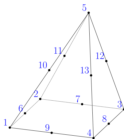
PYRA13
