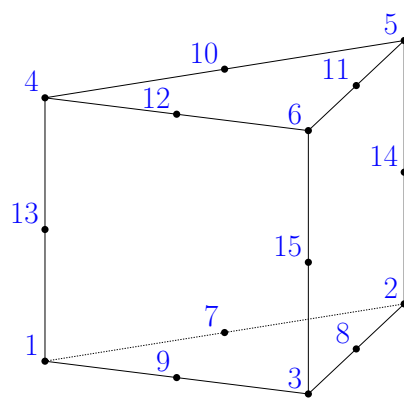
PENTA15
