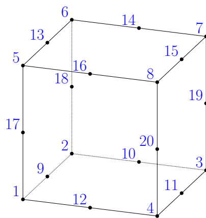
HEXA20
