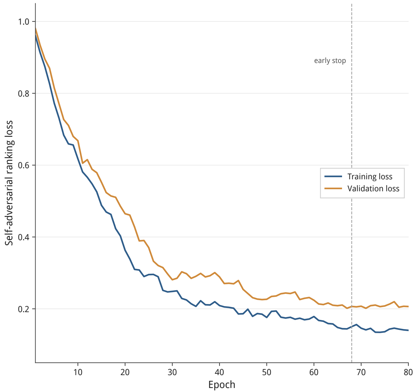
训练与验证损失曲线
