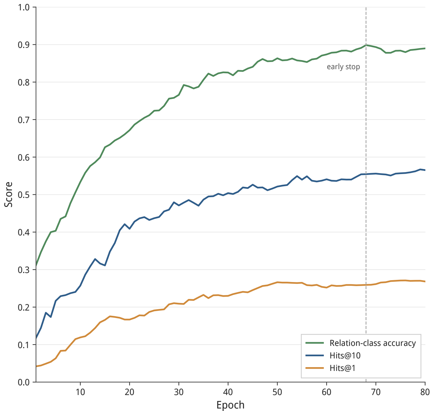
验证集准确率与排序指标曲线
