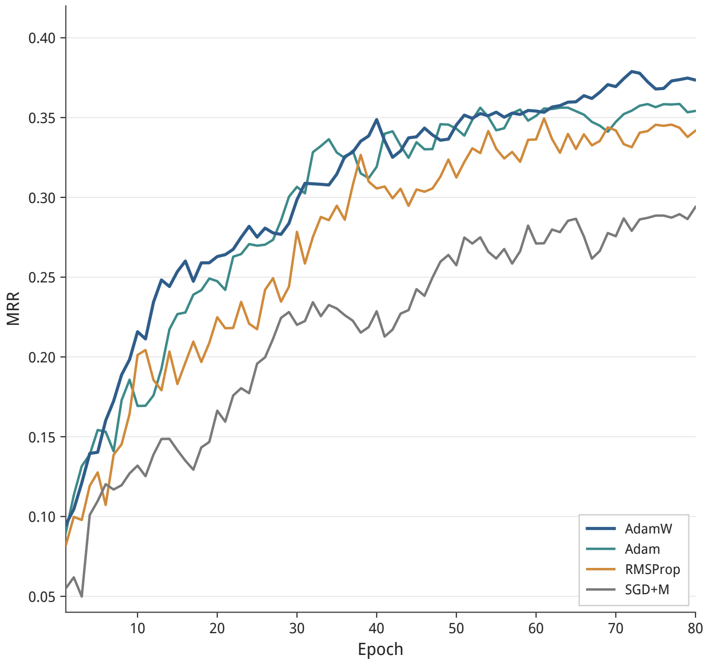
不同优化器的验证 MRR 对比
