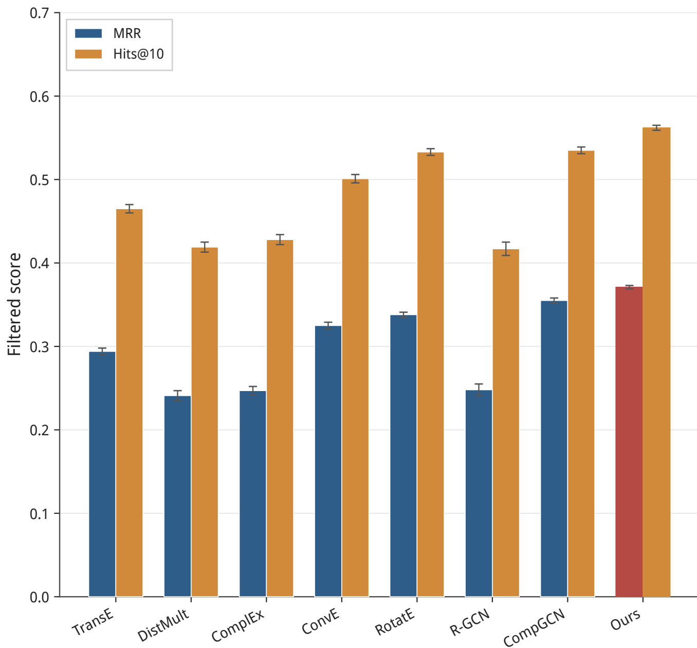
知识图谱嵌入模型性能对比
