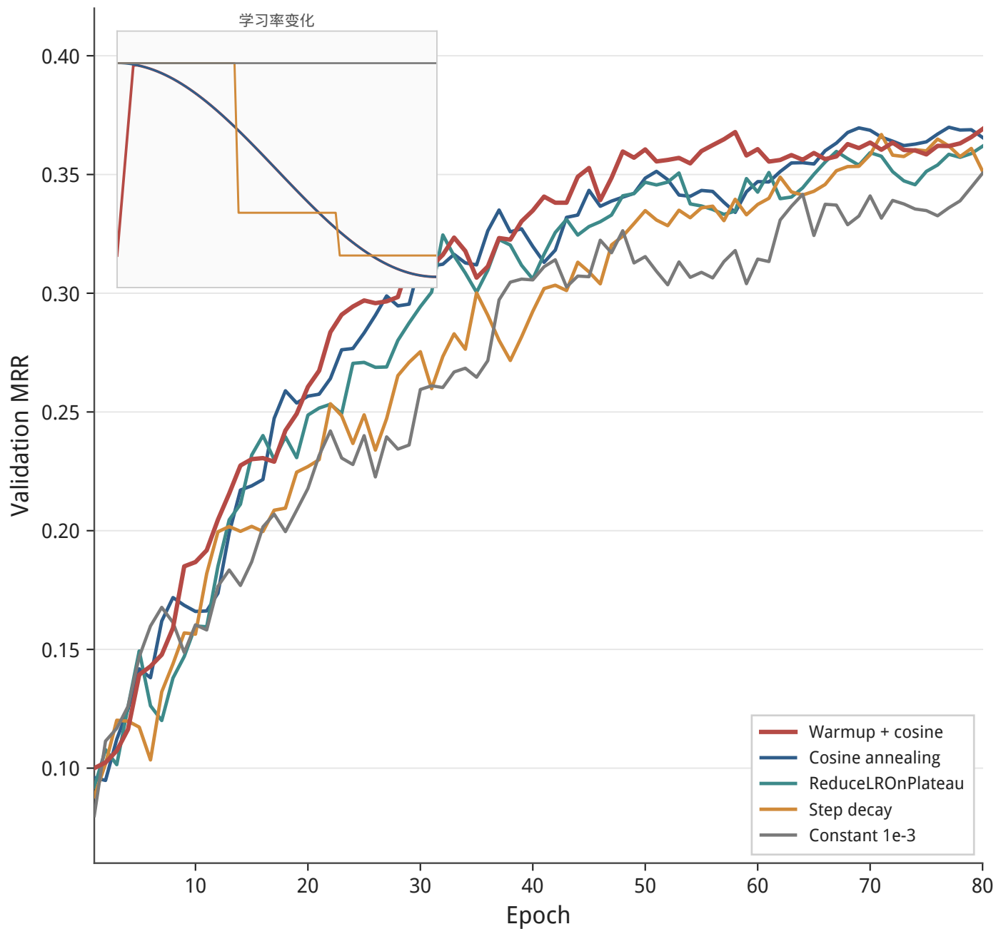
学习率策略对比
