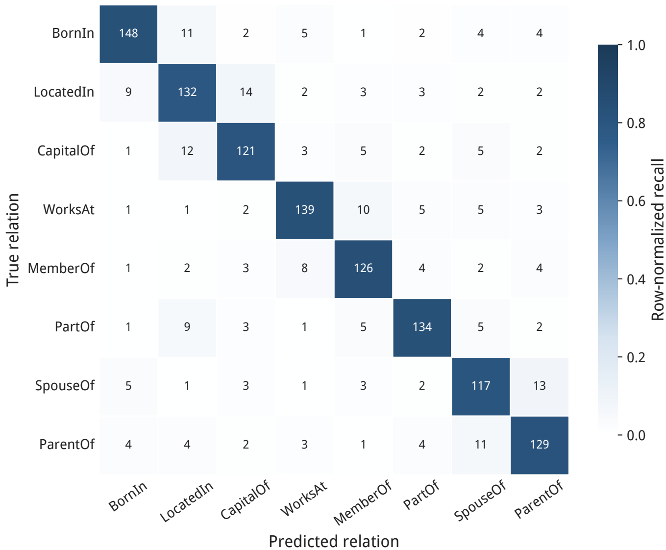
关系分类混淆矩阵
