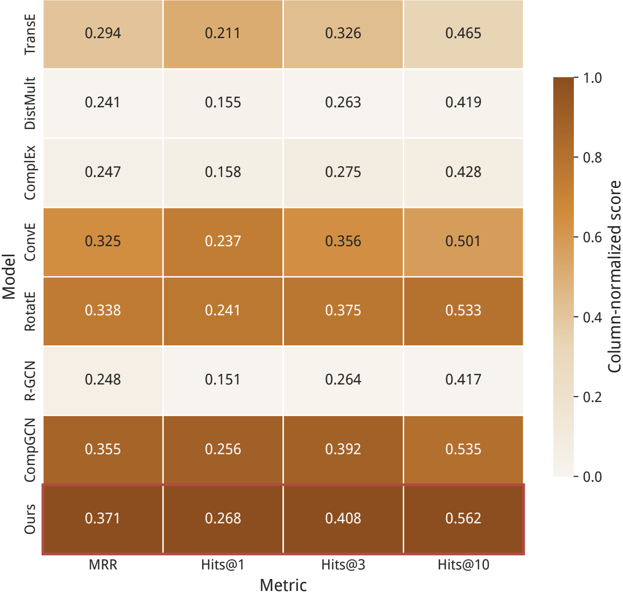
链接预测最终评测指标
