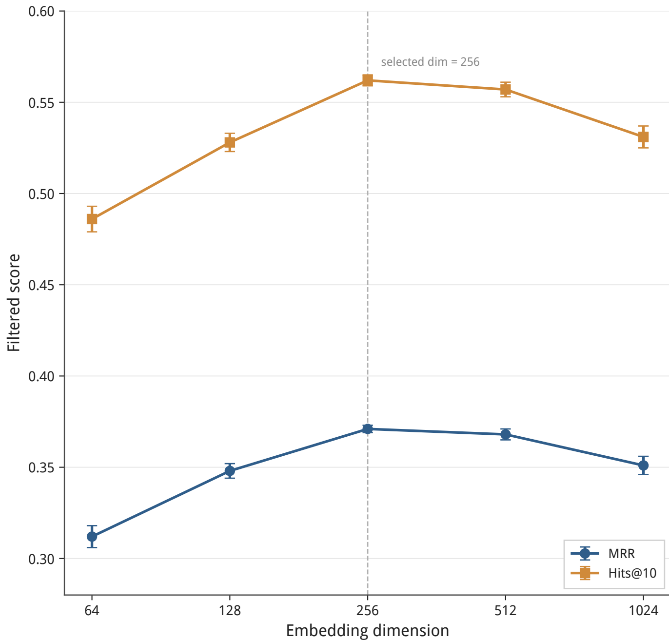
嵌入维度敏感性分析
