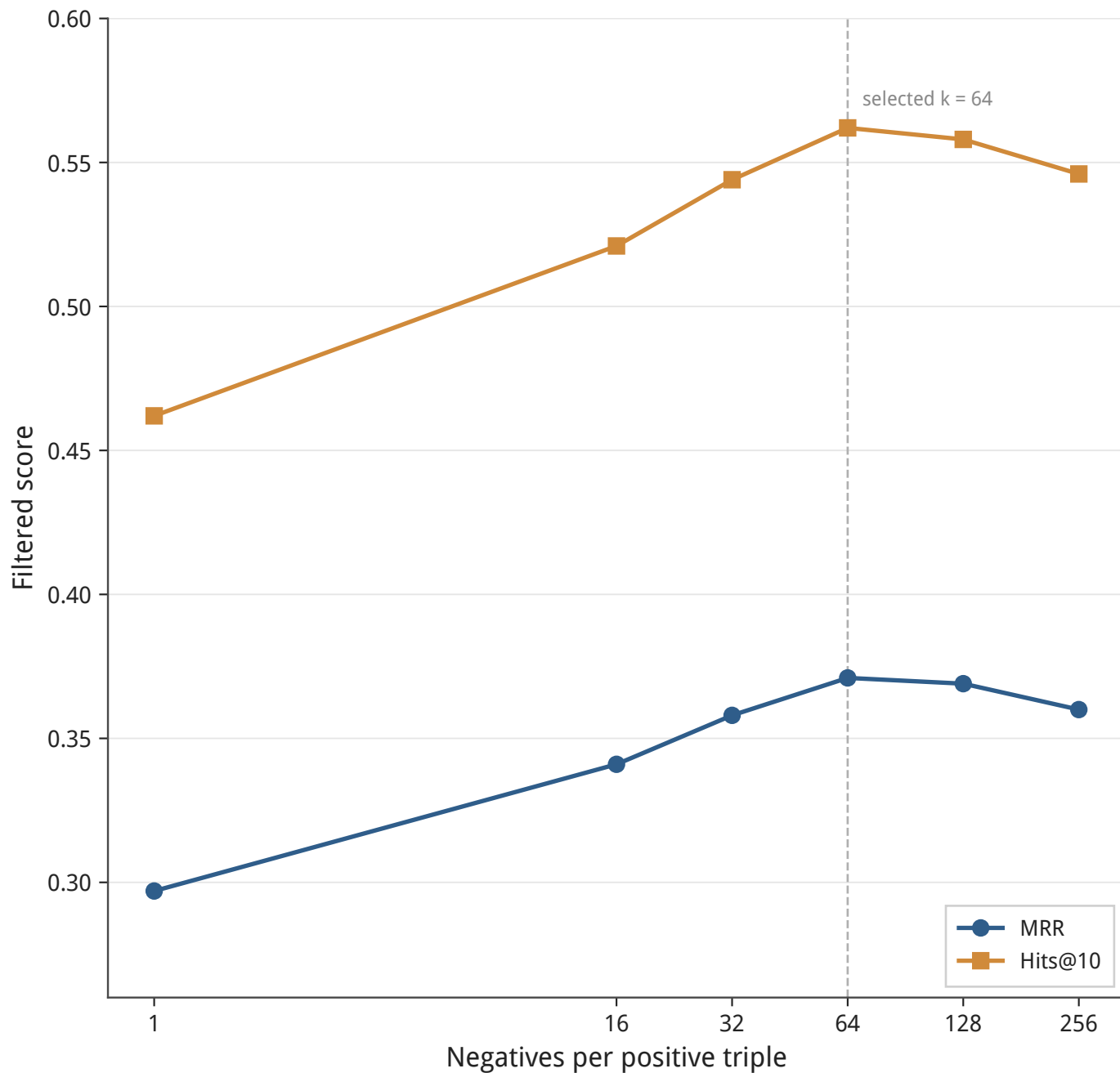
负采样数量的影响
