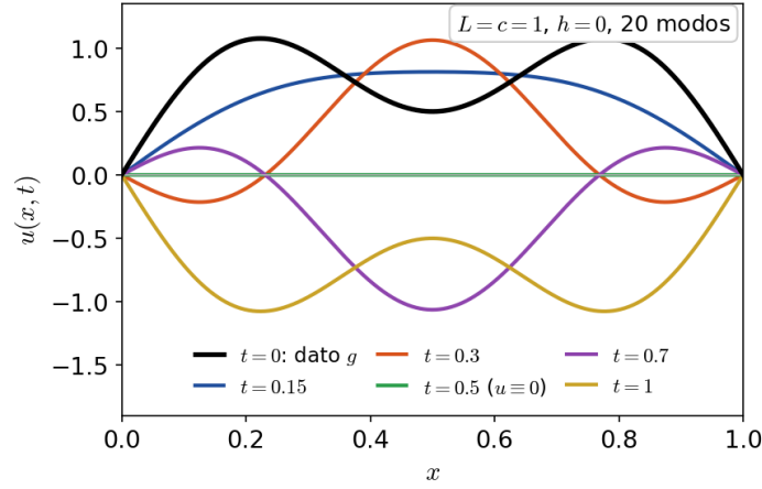
FIGURA 20.6. Solución de la ecuación de ondas con L = c = 1 , dato inicial g(x) = \sin \pi x + \frac{1}{2} \sin 3\pi x y h = 0 , en distintos instantes de tiempo. La serie se truncó a 20 modos, pero para este dato sólo A_1 = 1 y A_3 = \frac{1}{2} son no nulos, así que la figura muestra la solución exacta.
