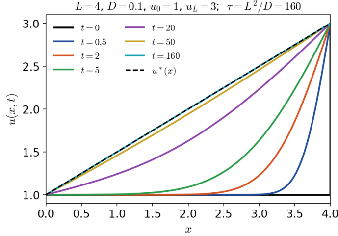
FIGURA 18.4. Evolución temporal de la solución u(x, t) de (18.3.1)-(18.3.2). En este ejemplo, L = 4 , D = 0,1 ; entonces L^2/D = 160 .
