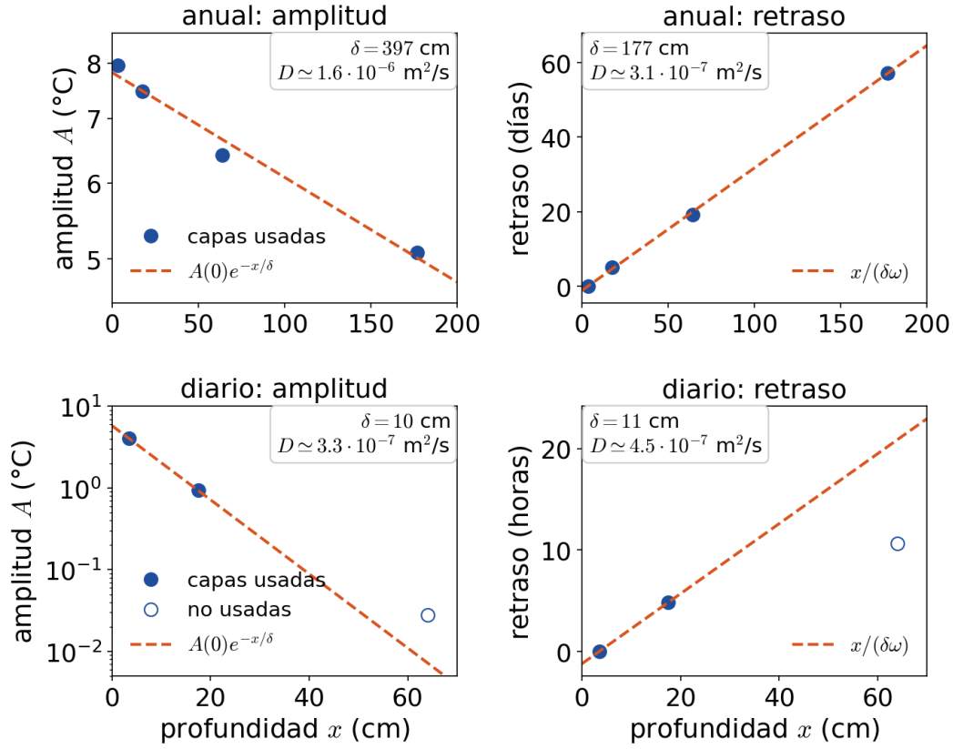
FIGURA 18.10. Estimación de la difusividad con los datos de la Figura 17.1: amplitud (escala logarítmica) y retraso de fase de los ciclos anual (arriba) y diario (abajo) en función de la profundidad media de cada capa, con las rectas -x/\delta ajustadas y el D = \delta^2\omega/2 resultante. Para el ciclo diario sólo se usan las dos capas superficiales; en la tercera el ciclo ya casi no se ve.
