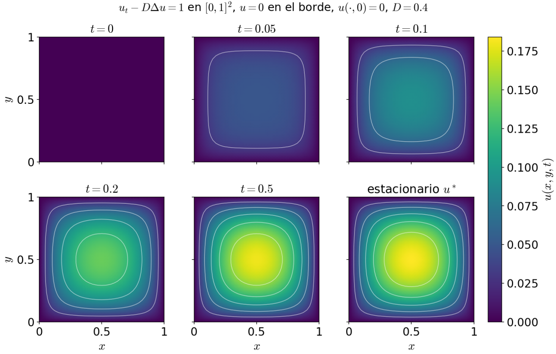
FIGURA 18.7. Solución de u_t - D\Delta u = 1 en [0, 1]^2 con u = 0 en el borde, u(\cdot, 0) = 0 y D = 0.4 , en varios instantes, y el estado estacionario u^* (misma escala de color). A t = 0.5 la diferencia con u^* es 2 \cdot 10^{-3} en norma L^2 .
