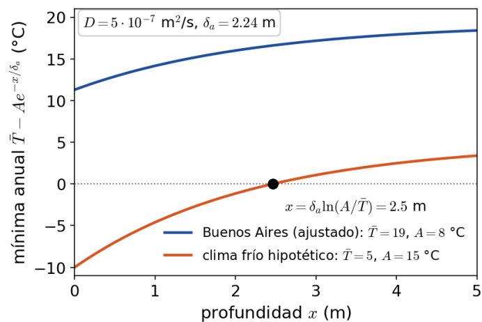
FIGURA 18.11. Temperatura mínima anual \bar{T} - Ae^{-x/\delta_a} en función de la profundidad, con D = 5 \cdot 10^{-7} \text{ m}^2/\text{s} ( \delta_a = 2,24 \text{ m} ). Con los valores ajustados para Buenos Aires ( \bar{T} = 19^\circ\text{C} , A = 8^\circ\text{C} ) el suelo no se congela ni en la superficie; en un clima frío hipotético ( \bar{T} = 5^\circ\text{C} , A = 15^\circ\text{C} ) hay que enterrar la cañería por debajo de x = \delta_a \ln(A/\bar{T}) \simeq 2,5 \text{ m} .
