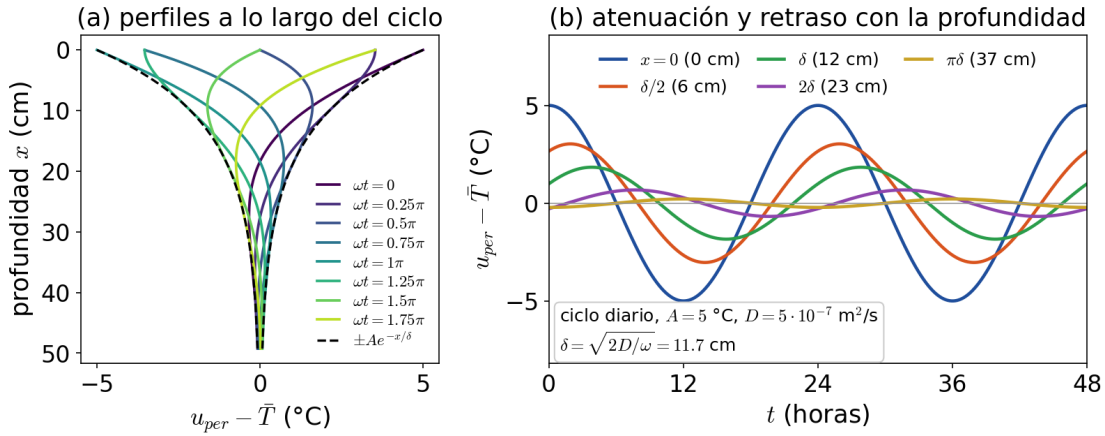
FIGURA 18.9. La solución periódica (18.6.2) para el ciclo diario con A = 5 \text{ °C} y D = 5 \cdot 10^{-7} \text{ m}^2/\text{s} ( \delta = 11,7 \text{ cm} ): (a) perfiles en profundidad a lo largo del ciclo, con la envolvente \pm Ae^{-x/\delta} ; (b) la oscilación a varias profundidades: atenuación e^{-x/\delta} y retraso x/(\delta\omega) ; a \pi\delta está en contrafase, con amplitud e^{-\pi}A .
