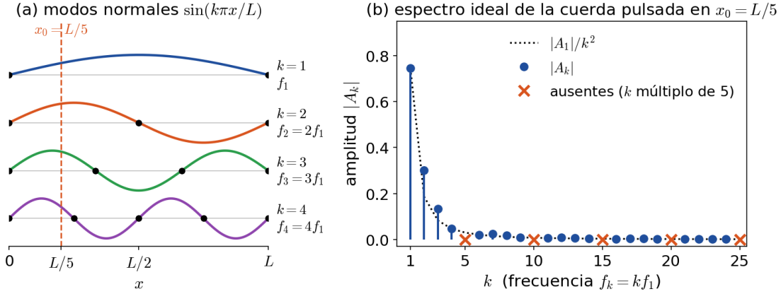
FIGURA 20.5. (a) Los primeros cuatro modos normales de la cuerda con extremos fijos y sus frecuencias f_k = kf_1 . (b) Espectro ideal de la cuerda pulsada en x_0 = L/5 : las amplitudes A_k decaen como 1/k^2 y faltan los armónicos múltiplos de 5, para los que x_0 es un nodo.
