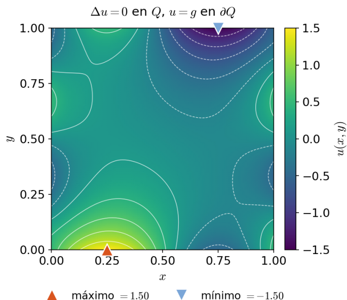
FIGURA 19.4. Solución de \Delta u = 0 en el cuadrado con u = g = \sin 2\pi x + \frac{1}{2} \cos 3\pi y en el borde: el máximo y el mínimo se alcanzan en \partial Q ; en el interior |u| < 1.43 .
