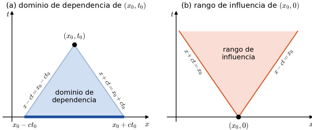
FIGURA 20.9. (a) Dominio de dependencia de (x_0, t_0) : u(x_0, t_0) sólo depende de los datos iniciales en [x_0 - ct_0, x_0 + ct_0] . (b) Rango de influencia de (x_0, 0) : el dato en x_0 sólo afecta a la solución en el cono |x - x_0| \leq ct .
