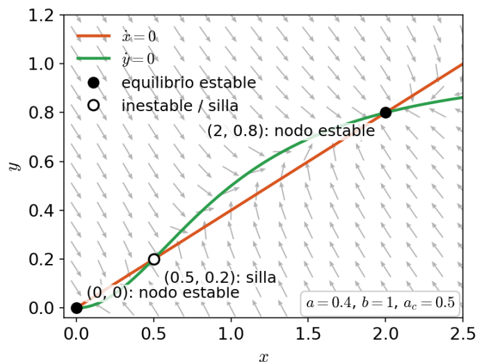
FIGURA 8.9. Gráfico de las nulclinas, equilibrios y campo vectorial en el caso a < a_c .
