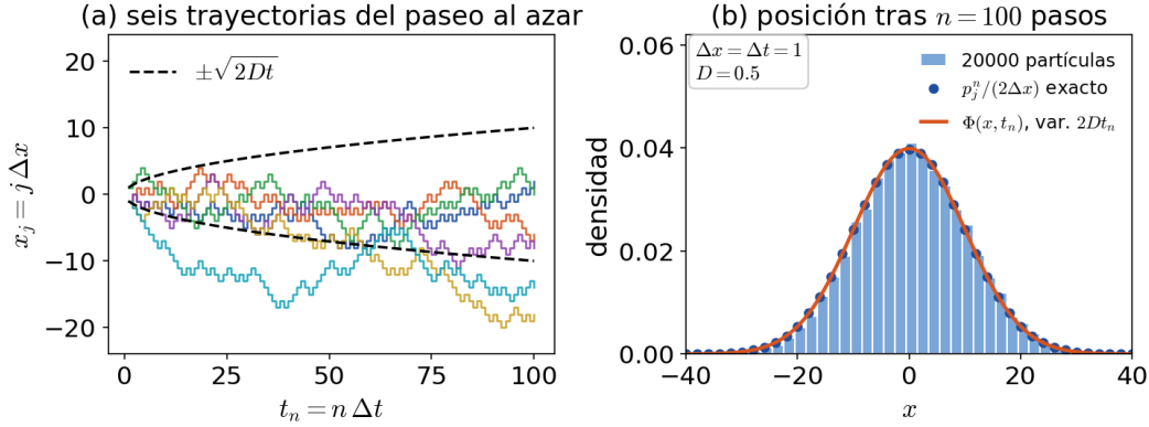
FIGURA 18.2. Paseo al azar simétrico con \Delta x = \Delta t = 1 ( D = 1/2 ): (a) trayectorias, con la envolvente \pm\sqrt{2Dt} ; (b) distribución de la posición tras n = 100 pasos comparada con la probabilidad exacta p_j^n y con la gaussiana de varianza n\Delta x^2 = 2Dt_n , la solución fundamental de la ecuación del calor.
