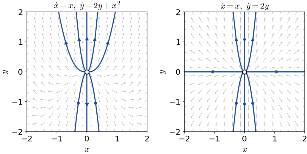
FIGURA 5.6. Los sistemas \dot{x} = x , \dot{y} = 2y + x^2 (izquierda) y su linealización \dot{x} = x , \dot{y} = 2y (derecha), con las mismas condiciones iniciales. Cerca del origen ambos son nodos inestables y el homeomorfismo \mathbf{h}(x, y) = (x, y - x^2 \ln |x|) lleva las trayectorias de uno en las del otro, pero ningún cambio de coordenadas de clase C^2 puede hacerlo.
