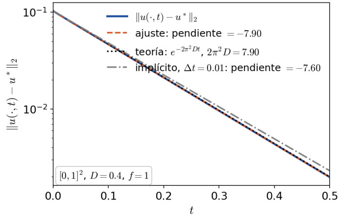
FIGURA 18.8. Gráfico semilogarítmico del error \|u(\cdot, t) - u^*\|_{L^2(\Omega)} para el ejemplo de la Figura 18.7, con la recta ajustada (pendiente -7.90 ) y la tasa teórica 2\pi^2 D . En gris, lo que da el esquema implícito con paso \Delta t = 0.01 : pendiente -7.60 .
