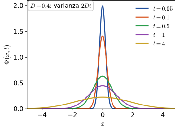
FIGURA 18.5. Distribución \Phi(x, t) para distintos valores de t .
