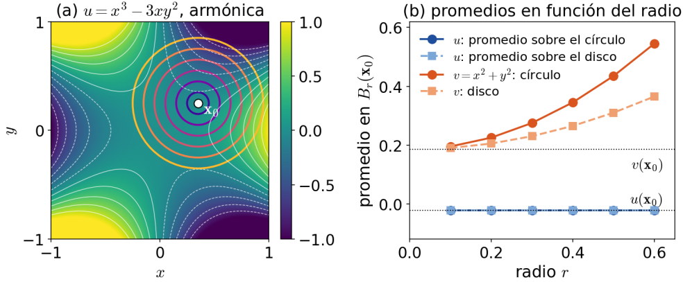
FIGURA 19.5. Propiedad del valor medio: para u = x^3 - 3xy^2 (armónica) el promedio sobre cualquier círculo o disco centrado en \mathbf{x}_0 es u(\mathbf{x}_0) ; para v = x^2 + y^2 , con \Delta v = 4 > 0 , el promedio sobre el círculo de radio r es v(\mathbf{x}_0) + r^2 y sobre el disco v(\mathbf{x}_0) + r^2/2 .
