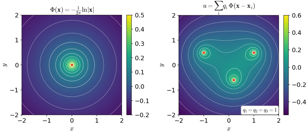
FIGURA 19.6. A la izquierda, solución fundamental del Laplaciano en dimensión 2 y a la derecha solución de la ecuación de Poisson asociada a tres cargas puntuales, obtenida por superposición de las soluciones fundamentales correspondientes.
