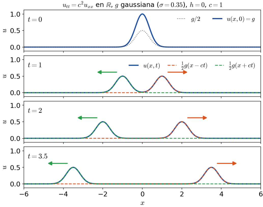
FIGURA 20.8. La fórmula de d'Alembert con h = 0 : el dato g se parte en dos mitades que viajan sin deformarse en sentidos opuestos con velocidad c .
