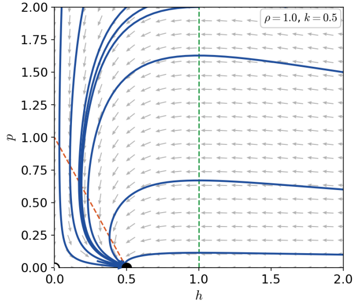
FIGURA 2.6. Diagrama de fases para el modelo (2.3.2) para k < 1 (en la figura, \rho = 1 y k = 0,5 ).
