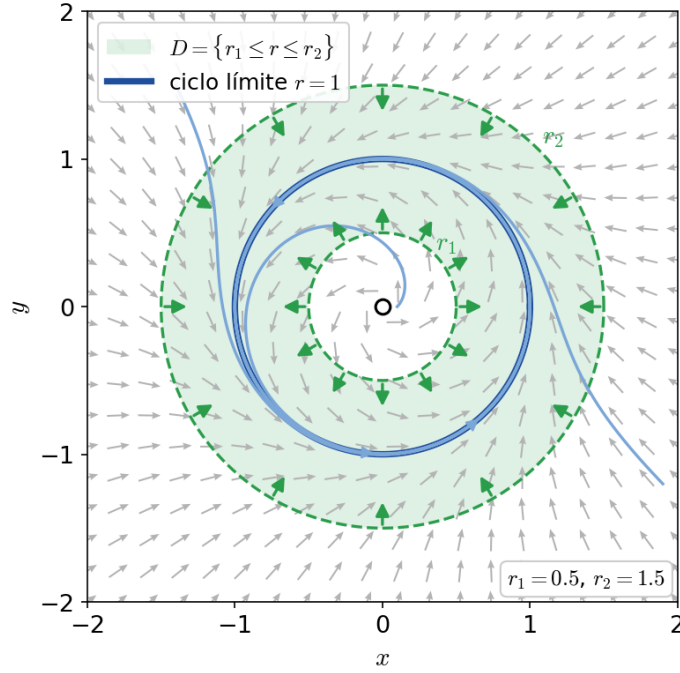
FIGURA 7.2. Diagrama de fases para el Ejemplo 7.2.3.
