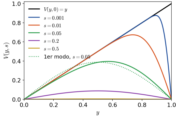
FIGURA 18.3. Evolución temporal del régimen transitorio V .
