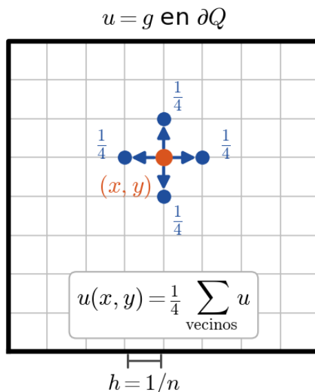
FIGURA 19.2. Interpretación probabilística de la ecuación de Laplace. El valor del juego en un punto interior es el promedio de los valores en los puntos vecinos, lo que en el límite continuo conduce a la ecuación \Delta u = 0 .
