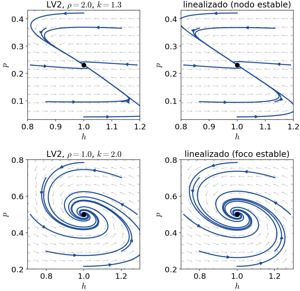
FIGURA 5.9. Hartman–Grobman en el modelo (2.3.2): a la izquierda el sistema en una ventana alrededor del equilibrio de coexistencia (1, 1 - 1/k) , a la derecha el sistema linealizado \dot{\mathbf{y}} = DF(\mathbf{x}^*)\mathbf{y} en las mismas coordenadas y con las mismas condiciones iniciales. Arriba \rho^2 \geq 4k(k-1) (nodo estable), abajo \rho^2 < 4k(k-1) (foco estable).
