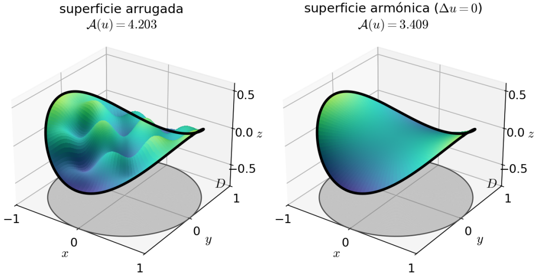
FIGURA 19.1. Dos superficies con el mismo borde (el alambre z = 0,3 \cos 2\theta sobre el disco unitario). A la izquierda, una superficie con ondulaciones interiores, de área 4,20; a la derecha, la gráfica de la función armónica con ese dato de borde, u = 0,3(x^2 - y^2) , de área 3,41.
