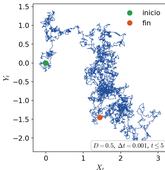
FIGURA 18.1. Realización de una partícula en un movimiento browniano ( D = 0,5 ).
