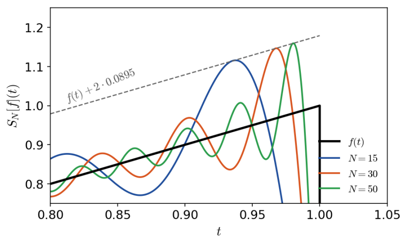
FIGURA 12.10. Fenómeno de Gibbs para la función diente de sierra.
