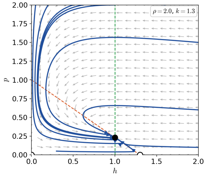
FIGURA 2.8. Diagrama de fases para el modelo (2.3.2) para k > 1 : acercamiento monótono al equilibrio de coexistencia (en la figura, \rho = 2 y k = 1,3 ).
