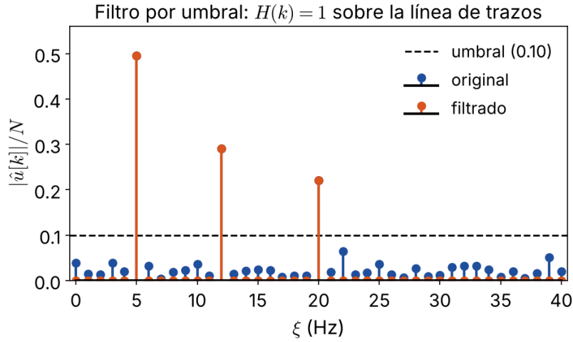
FIGURA 15.3. Filtro usado.
