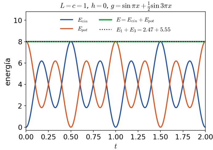
FIGURA 20.7. Energía cinética, energía potencial y energía total de la solución de la Figura 20.6; la total coincide con la suma por modos E_1 + E_3 de (20.4.1).
