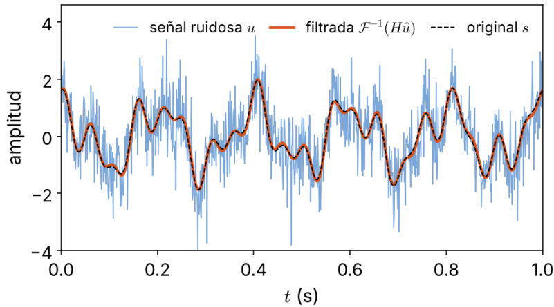
FIGURA 15.4. Señal filtrada.
