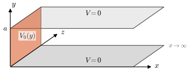
FIGURA 16.1. Ejercicio 16.2.13: dos placas a tierra en y = 0 e y = a , cerradas en x = 0 por una franja a potencial V_0(y) (problema adaptado de [17]).
