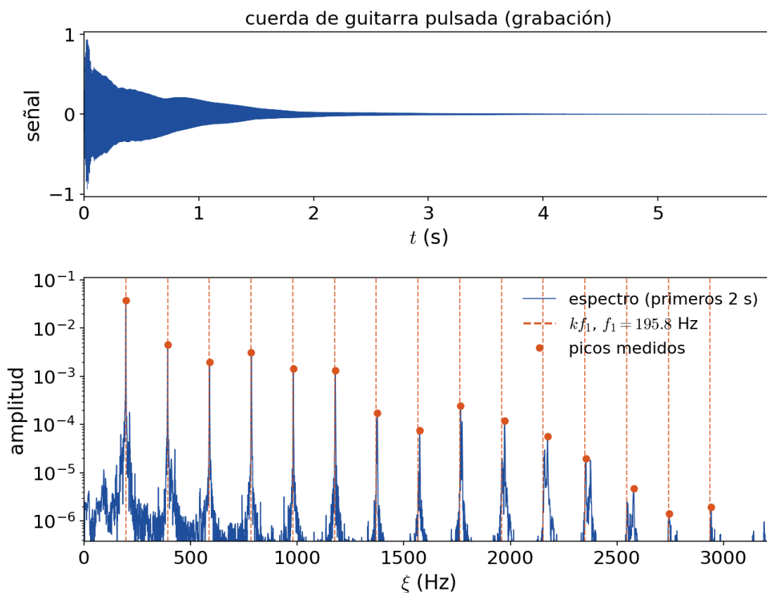
FIGURA 17.2. Grabación de una cuerda de guitarra pulsada (la tercera cuerda, Sol) y su espectro de amplitudes calculado con los primeros dos segundos. Las líneas de trazos marcan los múltiplos k f_1 de la fundamental medida, f_1 = 195,8 Hz: los picos están casi exactamente allí, pero el desvío crece con k (inarmónica) y las amplitudes de los armónicos altos son mucho menores. Los datos están en el repositorio de la materia (datos/cuerda_guitarra.wav).
