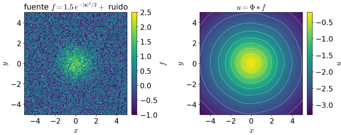
FIGURA 19.7. Fuente f ruidosa (izquierda) y solución de la ecuación de Poisson asociada (derecha) u = \Phi * f , ilustrando el efecto suavizante de la inversa del Laplaciano (la convolución con \Phi ).
