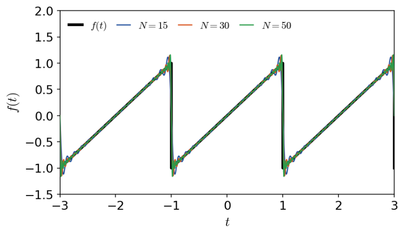
FIGURA 12.9. Función diente de sierra.
