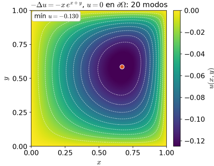
FIGURA 19.8. Aproximación de la solución de la ecuación de Poisson -\Delta u = f en (0, 1)^2 con condiciones de Dirichlet homogéneas mediante los modos k, \ell \leq 20 de la expansión en serie de Fourier. La fuente es f(x, y) = -x e^{x+y} ; el mínimo, -0,130 , se alcanza en (0,67, 0,59) .
