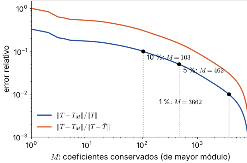
FIGURA 15.6. Error relativo de la reconstrucción de la serie de temperatura de 2023 conservando los M coeficientes de mayor módulo (calculado con Plancherel), en norma 2 respecto de \|T\| y de \|T - \bar{T}\| . Para un error relativo a \|T\| del 10 % alcanzan 103 coeficientes, para un 5 % hacen falta 462 y para un 1 %, 3662 de 8760.
