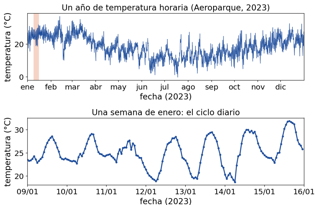
FIGURA 10.1. Un año de temperatura horaria del aire (Aeroparque, 2023; reanálisis ERA5 vía Open-Meteo) y detalle de una semana de enero, donde se ve el ciclo diario superpuesto a la variabilidad irregular.
