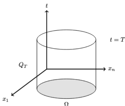
FIGURA 18.6. Cilindro espacio-temporal Q_T = \Omega \times (0, T] .
