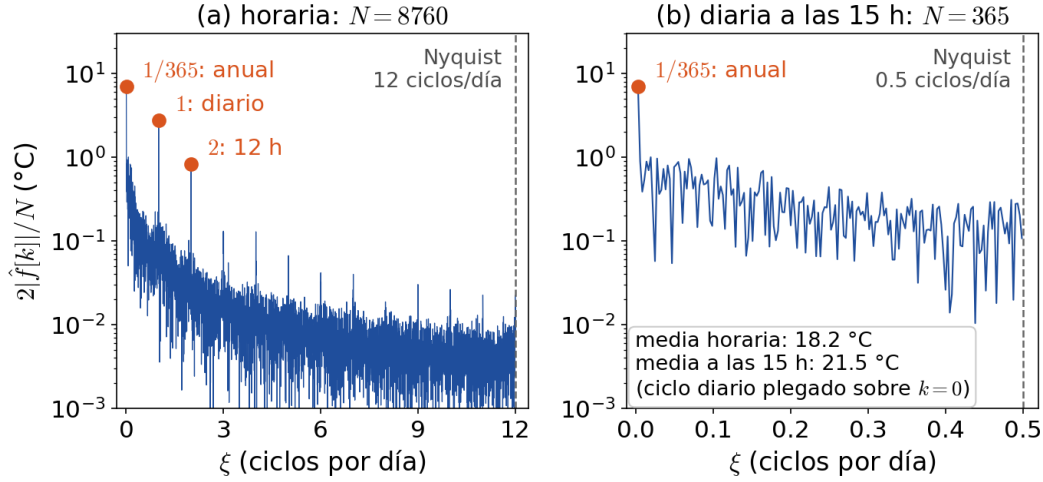
FIGURA 14.3. (a) Espectro de amplitudes de la temperatura horaria de 2023 en ciclos por día, hasta la frecuencia de Nyquist (12 ciclos/día); se marcan el ciclo anual (1/365), el diario (1) y su armónico de 12 h (2). (b) Espectro de la misma señal muestreada una vez por día a las 15 h: la frecuencia de Nyquist baja a 0,5 ciclos/día, el ciclo anual sigue intacto y el diario se pliega sobre k = 0 : la media sube de 18,2 a 21,5 °C.
