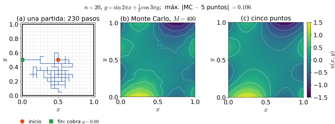
FIGURA 19.3. El juego con n = 20 y pago g = \sin 2\pi x + \frac{1}{2} \cos 3\pi y en el borde: (a) una partida desde el centro; (b) el valor esperado estimado promediando 400 partidas desde cada nodo; (c) la solución exacta de la ecuación de promedios. La diferencia entre (b) y (c) (error cuadrático medio 0,03, máximo 0,11) es el ruido estadístico, del orden de \sigma/\sqrt{M} .
