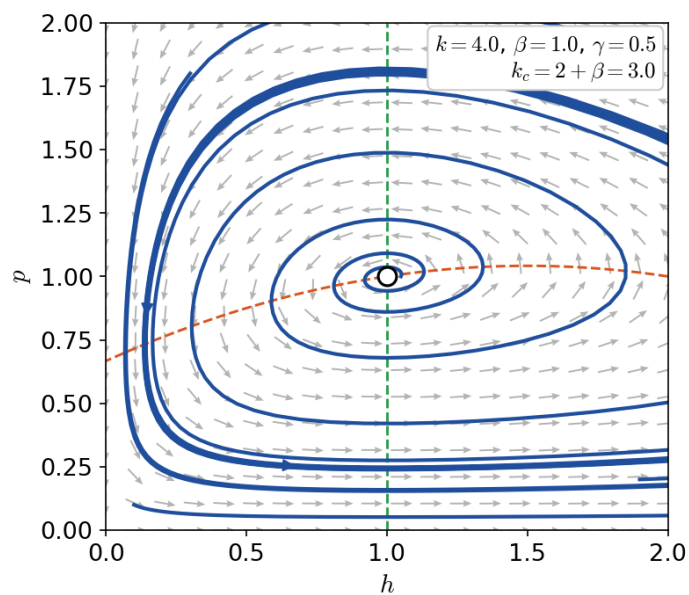
FIGURA 2.11. Aparición de un ciclo límite en el sistema (2.4.2) cuando k > k_c (en la figura, k = 4 , \beta = 1 y \gamma = 0,5 ).
