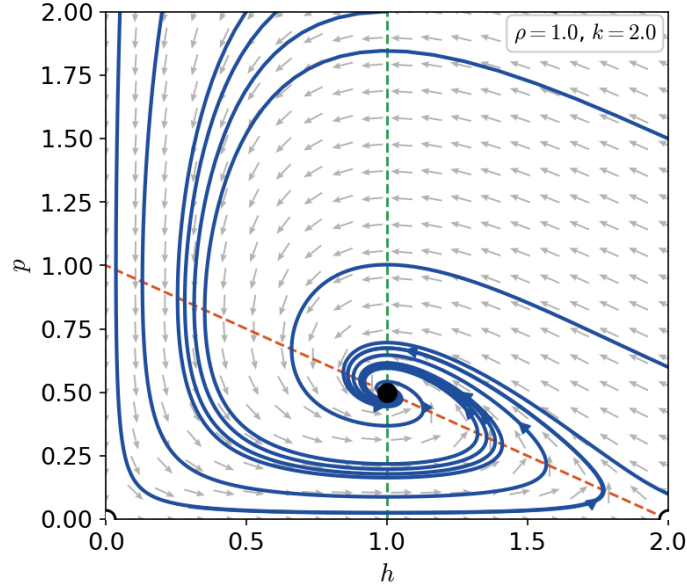
FIGURA 2.9. Diagrama de fases para el modelo (2.3.2) para k > 1 : acercamiento oscilatorio al equilibrio de coexistencia (en la figura, \rho = 1 y k = 2 ).
