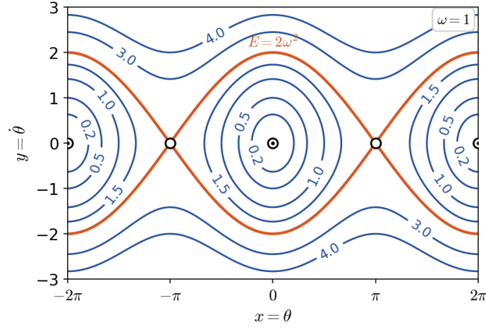
FIGURA 6.1. Curvas de nivel para la energía asociada al péndulo simple.
