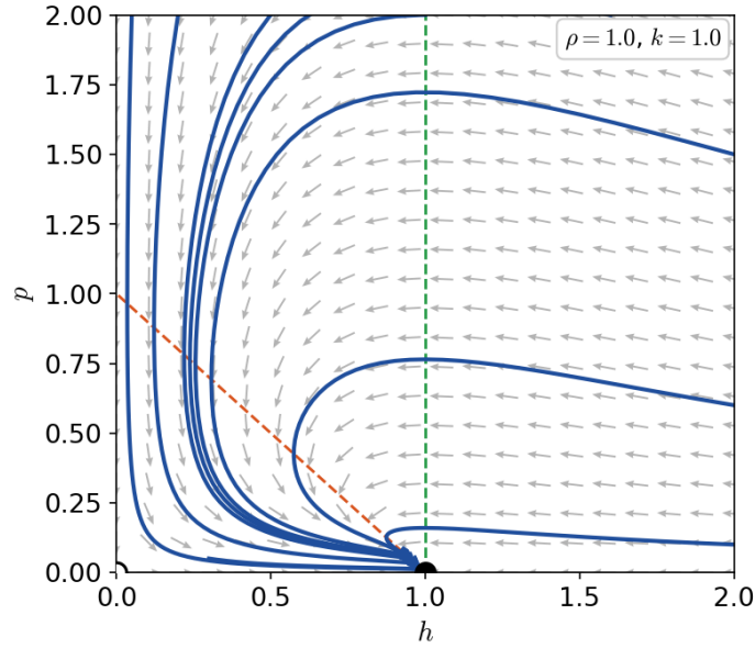
FIGURA 2.7. Diagrama de fases para el modelo (2.3.2) para k = 1 (en la figura, \rho = 1 ).
