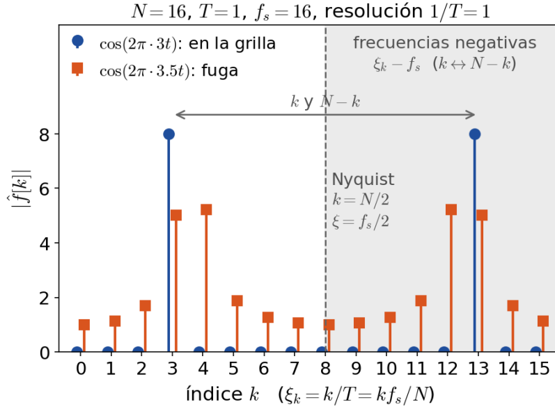
FIGURA 14.2. Grilla de frecuencias de la DFT con N = 16 , T = 1 ( f_s = 16 ). |\hat{f}[k]| para \cos(2\pi \cdot 3t) , cuya frecuencia cae en la grilla (dos picos, k = 3 y N - k = 13 ), y para \cos(2\pi \cdot 3.5t) , que cae entre dos puntos y reparte su energía en todos los índices (fuga espectral). Los índices k > N/2 son las frecuencias negativas \xi_k - f_s ; la línea punteada es la frecuencia de Nyquist.
