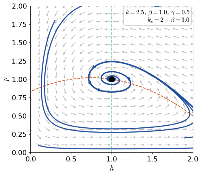
FIGURA 2.10. Diagrama de fases para el modelo (2.4.2) cuando k < k_c : las trayectorias convergen al equilibrio (1, 1) (en la figura, k = 2,5 , \beta = 1 y \gamma = 0,5 ).
