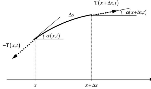
FIGURA 20.4. Tensión en los puntos extremos de un segmento pequeño de una cuerda.
