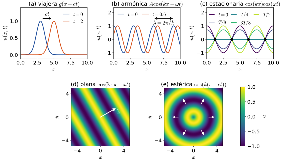
FIGURA 20.2. Catálogo de ondas: (a) onda viajera g(x - ct) : el perfil se traslada rígidamente; (b) onda armónica A \cos(kx - \omega t) ; (c) onda estacionaria 2A \cos(kx) \cos(\omega t) : los nodos no se mueven; (d) onda plana en el plano: frentes rectos perpendiculares a \mathbf{k} ; (e) onda esférica: frentes circulares. Los dos mapas de color comparten la escala.
