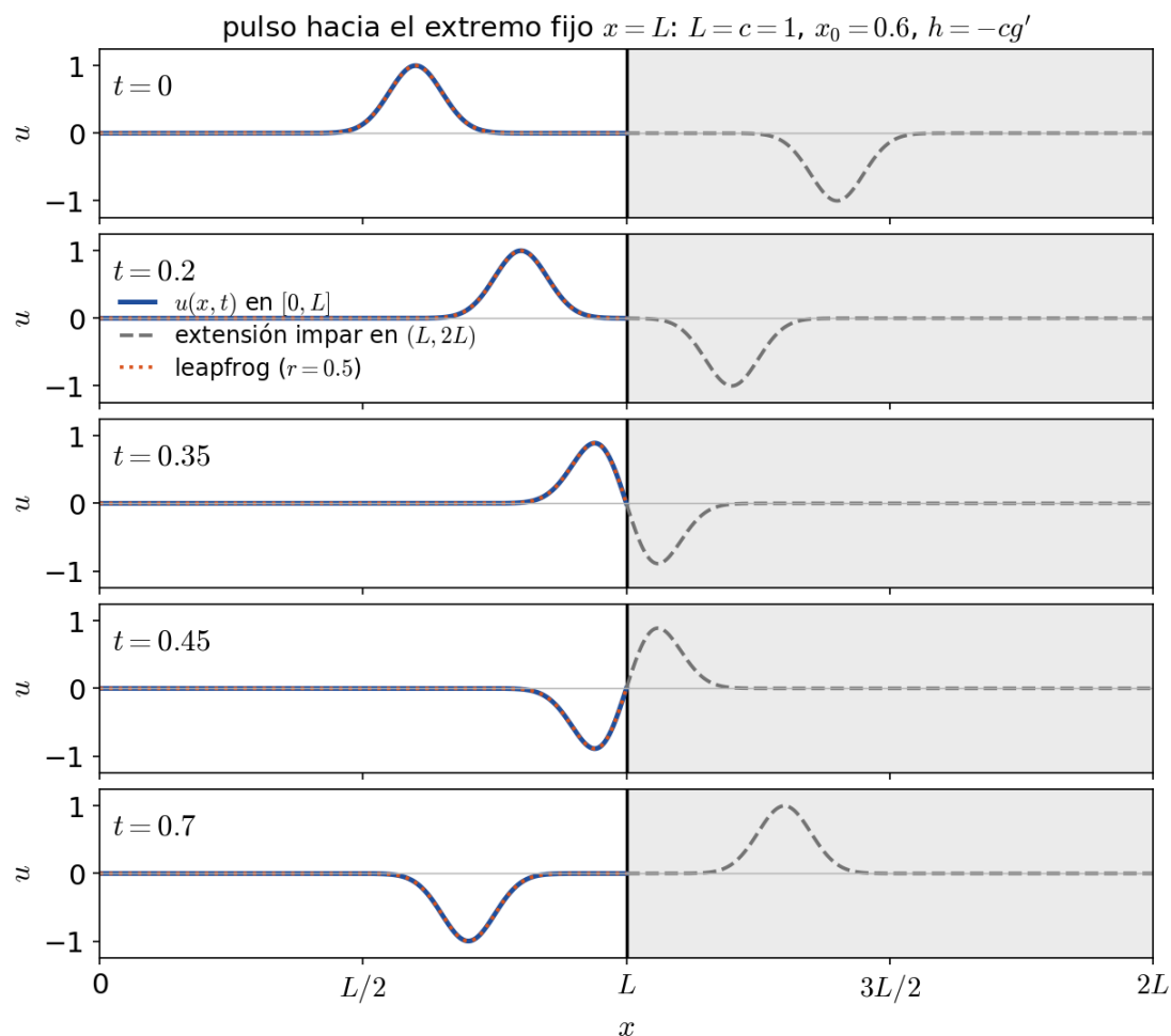
FIGURA 20.10. Reflexión de un pulso en el extremo fijo x = L ( L = c = 1 ). En [0, L] , la solución; en (L, 2L) , sombreada, la extensión impar del dato: la “imagen” invertida viaja hacia la izquierda y entra en [0, L] cuando el pulso sale, de modo que el pulso vuelve invertido. En el instante en que el pulso y su imagen se superponen la cuerda está momentáneamente plana y toda la energía es cinética. Superpuesta a la solución exacta, la aproximación del esquema numérico leapfrog (Ejercicio 21.2.10) con r = c\Delta t/\Delta x = 0.5 .
