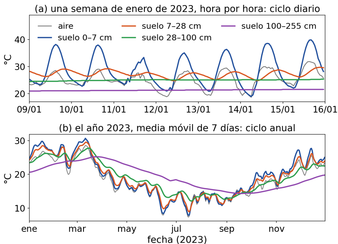
FIGURA 17.1. Temperatura del aire y del suelo en cuatro capas (0–7, 7–28, 28–100 y 100–255 cm; reanálisis ERA5-Land para Aeroparque, 2023): (a) una semana de enero, hora por hora: el ciclo diario se atenúa y se retrasa con la profundidad, y a 28–100 cm ya desaparece; (b) el año en medias móviles de 7 días: el ciclo anual se atenúa mucho menos y llega a la capa más profunda con casi dos meses de retraso. Los datos están en el repositorio de la materia ( datos/suelo_horaria.csv ).
