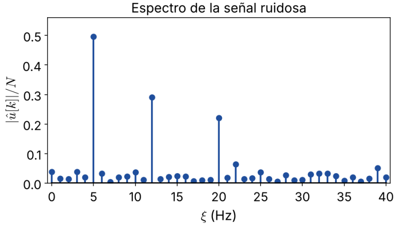
FIGURA 15.2. Análisis espectral de la señal ruidosa.
