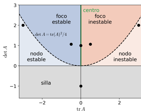
FIGURA 5.5. Regiones descritas en el Teorema 5.2.3.
