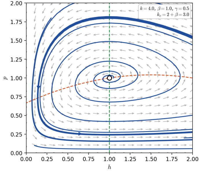
FIGURA 2.10. Aparición de un ciclo límite en el sistema (2.4.2) cuando k > k_c .
