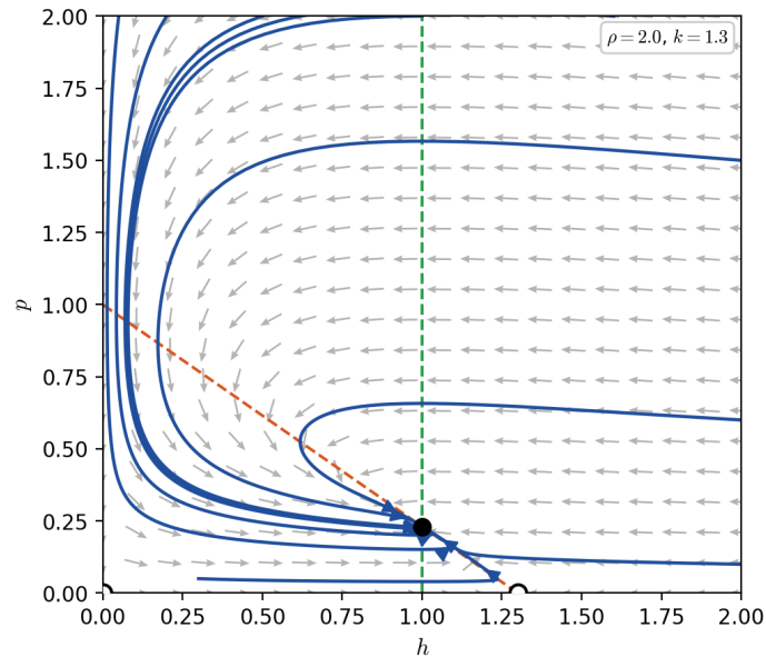
FIGURA 2.7. Diagrama de fases para el modelo (2.3.2) para k > 1 : acercamiento monótono al equilibrio de coexistencia (en la figura, k = 1,3 ).
