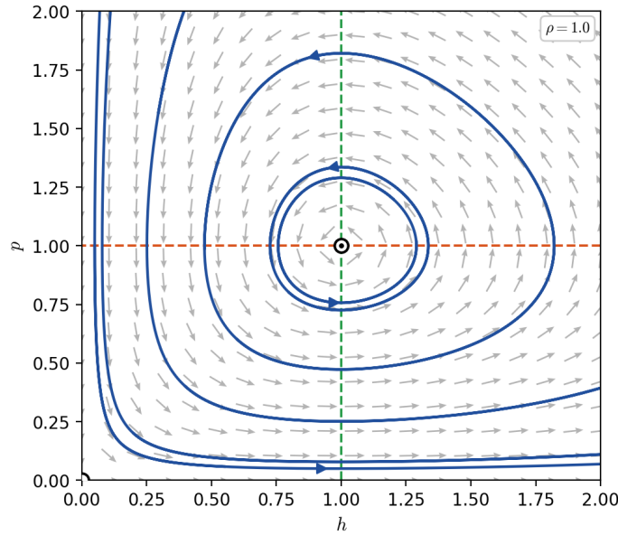
FIGURA 2.4. Diagrama de fases para el modelo (2.2.1). Los ejes corresponden a h (horizontal) y p (vertical). Las trayectorias son las curvas de nivel de \mathcal{H} .
