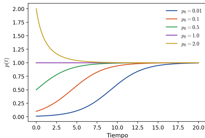
FIGURA 2.3. Solución de la ecuación logística para diferentes condiciones iniciales.
