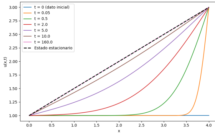
FIGURA 18.3. Evolución temporal la solución u(x, t) de (18.3.1)-(18.3.2). En este ejemplo, L = 4 , D = 0,1 ; entonces L^2/D = 160 .
