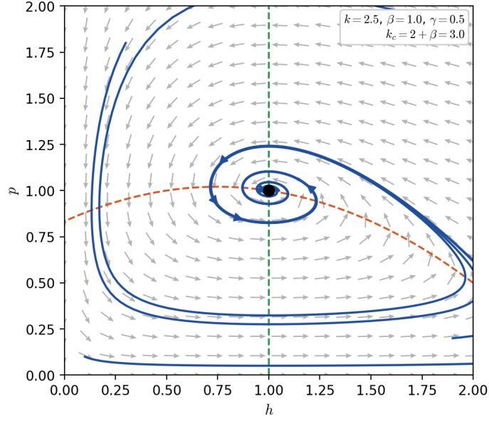
FIGURA 2.9. Diagrama de fases para el modelo (2.4.2) cuando k < k_c : las trayectorias convergen al equilibrio (1, 1) .
