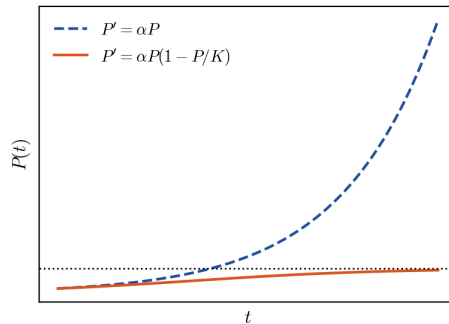
FIGURA 2.2. Comparación entre el modelo malthusiano y el modelo logístico.
