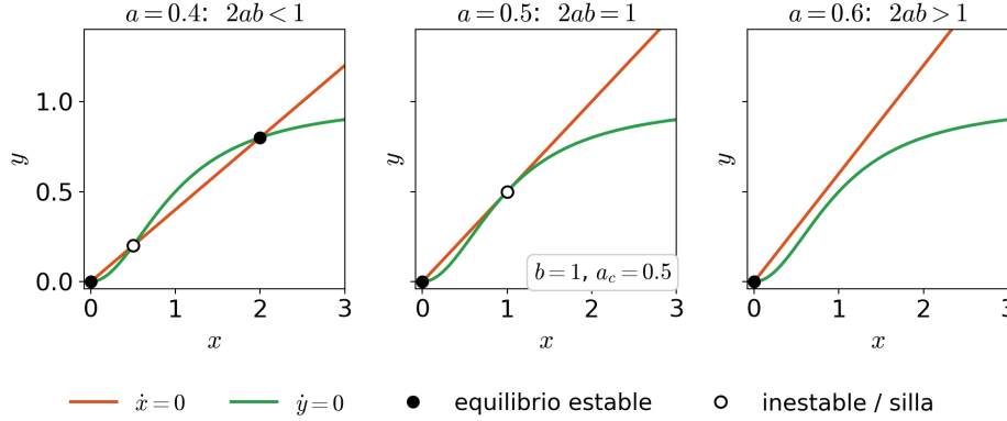
FIGURA 8.8. Gráfico de las nulclinas para el sistema (8.4.1).
