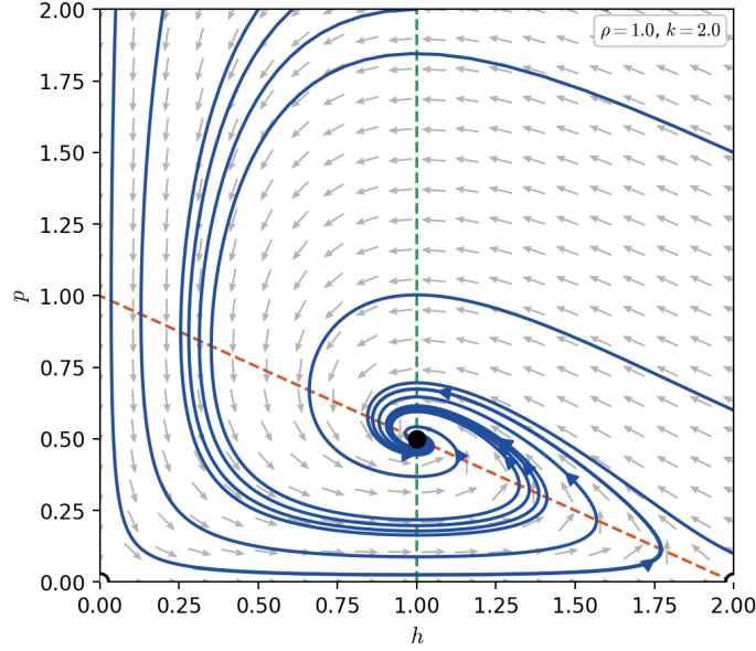
FIGURA 2.8. Diagrama de fases para el modelo (2.3.2) para k > 1 : acercamiento oscilatorio al equilibrio de coexistencia (en la figura, k = 2 ).
