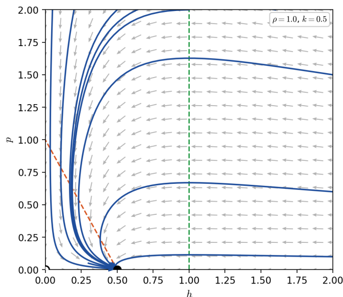
FIGURA 2.5. Diagrama de fases para el modelo (2.3.2) para k < 1 (en la figura, k = 0.5 ).
