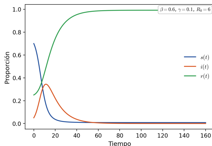
FIGURA 2.11. Evolución temporal del modelo SIR con datos iniciales s(0) = 0,7 , i(0) = 0,05 , r(0) = 0,25 y parámetros \beta = 0,6 y \gamma = 0,1 ( R_0 = 6 ).
