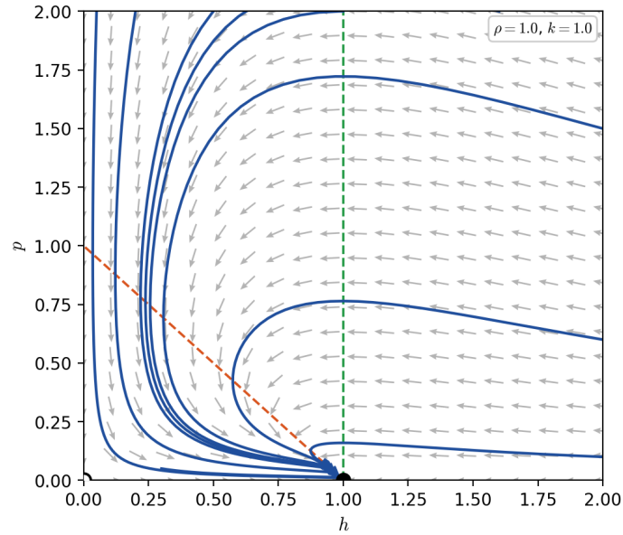
FIGURA 2.6. Diagrama de fases para el modelo (2.3.2) para k = 1 .
