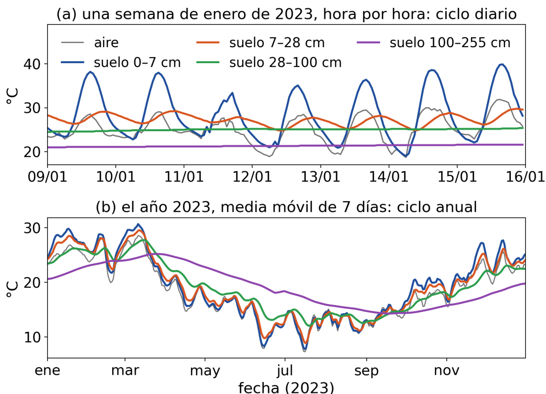
FIGURA 17.1. Temperatura del aire y del suelo en cuatro capas (0–7, 7–28, 28–100 y 100–255 cm; reanálisis ERA5-Land para Aeroparque, 2023): (a) una semana de enero, hora por hora: el ciclo diario se atenúa y se retrasa con la profundidad, y a 28–100 cm ya desaparece; (b) el año en medias móviles de 7 días: el ciclo anual se atenúa mucho menos y llega a la capa más profunda con casi dos meses de retraso. Los datos están en el repositorio de la materia ( datos/suelo_horaria.csv ).
