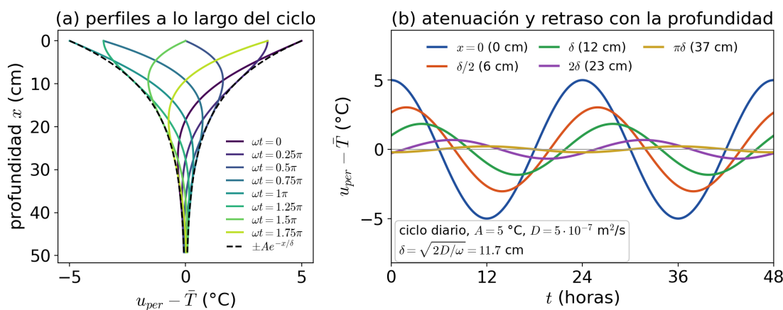
FIGURA 18.9. La solución periódica (18.6.2) para el ciclo diario con A = 5 \text{ }^\circ\text{C} y D = 5 \cdot 10^{-7} \text{ m}^2/\text{s} ( \delta = 11,7 \text{ cm} ): (a) perfiles en profundidad a lo largo del ciclo, con la envolvente \pm Ae^{-x/\delta} ; (b) la oscilación a varias profundidades: atenuación e^{-x/\delta} y retraso x/(\delta\omega) ; a \pi\delta está en contrafase, con amplitud e^{-\pi}A .
