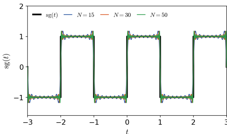
FIGURA 12.7. Fenómeno de Gibbs para la función signo.
