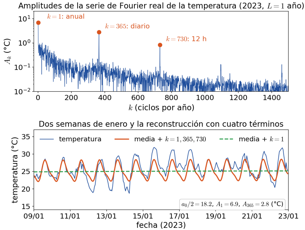
FIGURA 11.4. Serie de Fourier real de la temperatura de 2023 ( L = 1 año). Arriba: amplitudes A_k ; sobresalen el ciclo anual ( k = 1 , A_1 \approx 6,9 ^{\circ}\text{C} ), el diario ( k = 365 , A_{365} \approx 2,8 ^{\circ}\text{C} ) y su primer armónico ( k = 730 ). Abajo: dos semanas de enero y la reconstrucción con sólo la media y esos tres términos, que explican el 70 % de la varianza.
