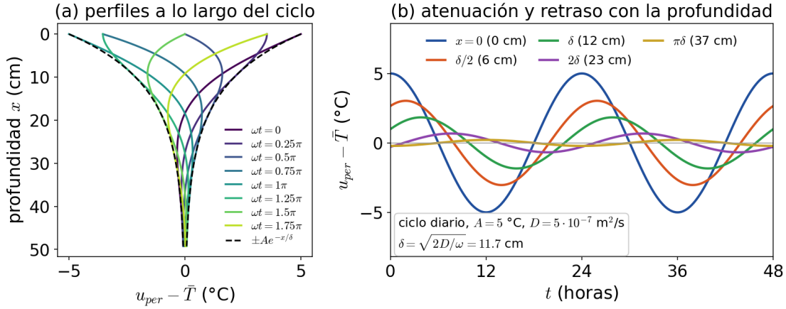
FIGURA 18.9. La solución periódica (18.6.2) para el ciclo diario con A = 5 °C y D = 5 \cdot 10^{-7} m 2 /s ( \delta = 11,7 cm): (a) perfiles en profundidad a lo largo del ciclo, con la envolvente \pm Ae^{-x/\delta} ; (b) la oscilación a varias profundidades: atenuación e^{-x/\delta} y retraso x/(\delta\omega) ; a \pi\delta está en contrafase, con amplitud e^{-\pi}A .
