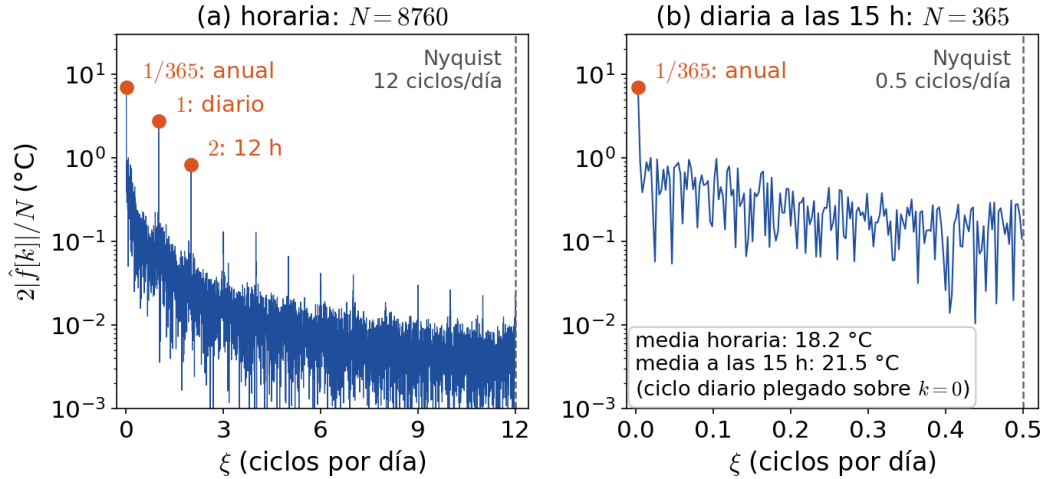
FIGURA 14.3. (a) Espectro de amplitudes de la temperatura horaria de 2023 en ciclos por día, hasta la frecuencia de Nyquist (12 ciclos/día); se marcan el ciclo anual ( 1/365 ), el diario (1) y su armónico de 12 h (2). (b) Espectro de la misma señal muestreada una vez por día a las 15 h: la frecuencia de Nyquist baja a 0,5 ciclos/día, el ciclo anual sigue intacto y el diario se pliega sobre k = 0 : la media sube de 18,2 a 21,5 °C.
