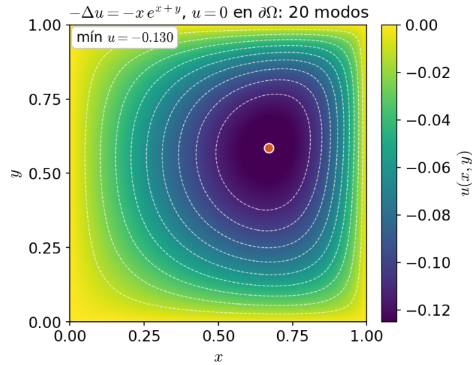
FIGURA 19.8. Aproximación de la solución de la ecuación de Poisson -\Delta u = f con condiciones de Dirichlet homogéneas mediante los primeros 20 modos de la expansión en serie de Fourier. La fuente es f(x, y) = -x e^{x+y} ; el mínimo, -0,130 , se alcanza en (0,67, 0,59) .
