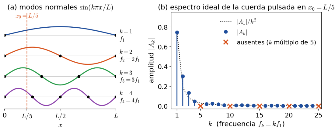
FIGURA 20.5. (a) Los primeros cuatro modos normales de la cuerda con extremos fijos y sus frecuencias f_k = kf_1 . (b) Espectro ideal de la cuerda pulsada en x_0 = L/5 : las amplitudes A_k decaen como 1/k^2 y faltan los armónicos múltiplos de 5, para los que x_0 es un nodo.
