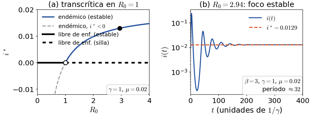
FIGURA 8.14. SIR con nacimientos (8.6.1), \gamma = 1 , \mu = 0,02 . (a) Diagrama de bifurcación: la rama endémica i^* = \frac{\mu}{\beta}(R_0 - 1) intercambia estabilidad con la libre de enfermedad en R_0 = 1 ; el punto lleno es el equilibrio del panel (b). (b) Con \beta = 3 ( R_0 \approx 2,94 ) el equilibrio endémico es un foco estable: i(t) se acerca a i^* con ondas de período \approx 32 (escala logarítmica).
