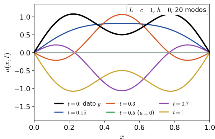
FIGURA 20.6. Solución de la ecuación de ondas con L = c = 1 , dato inicial g(x) = \sin \pi x + \frac{1}{2} \sin 3\pi x y h = 0 , en distintos instantes de tiempo (para este dato la serie tiene sólo dos términos).
