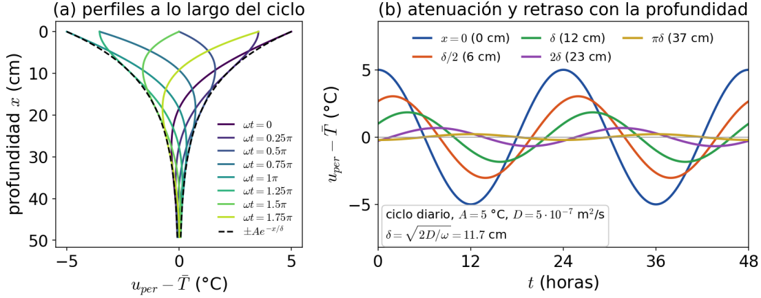
FIGURA 18.9. La solución periódica (18.6.2) para el ciclo diario con A = 5 \text{ } ^\circ\text{C} y D = 5 \cdot 10^{-7} \text{ m}^2/\text{s} ( \delta = 11,7 \text{ cm} ): (a) perfiles en profundidad a lo largo del ciclo, con la envolvente \pm Ae^{-x/\delta} ; (b) la oscilación a varias profundidades: atenuación e^{-x/\delta} y retraso x/(\delta\omega) ; a \pi\delta está en contrafase, con amplitud e^{-\pi}A .
