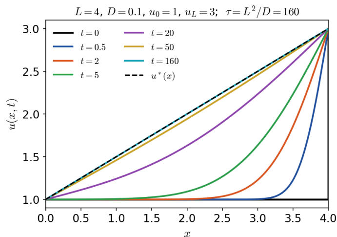
FIGURA 18.4. Evolución temporal la solución u(x, t) de (18.3.1)-(18.3.2). En este ejemplo, L = 4 , D = 0,1 ; entonces L^2/D = 160 .
