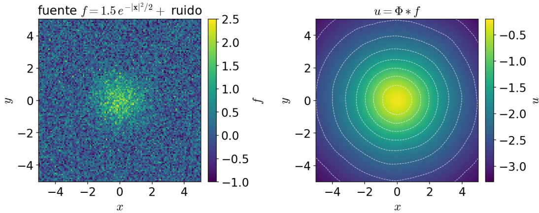
FIGURA 19.7. Fuente f ruidosa (izquierda) y solución de la ecuación de Poisson asociada (derecha) u = \Phi * f , ilustrando el efecto suavizante del operador Laplaciano.
